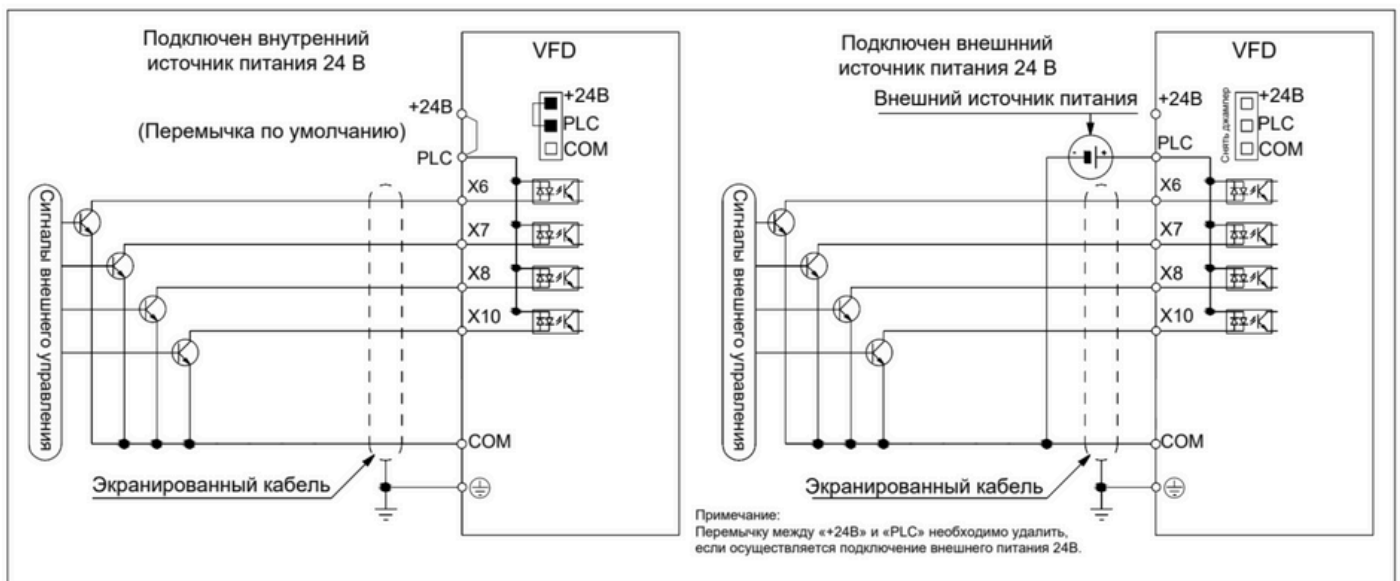
Рис. 2.1.1 Подключение NPN
