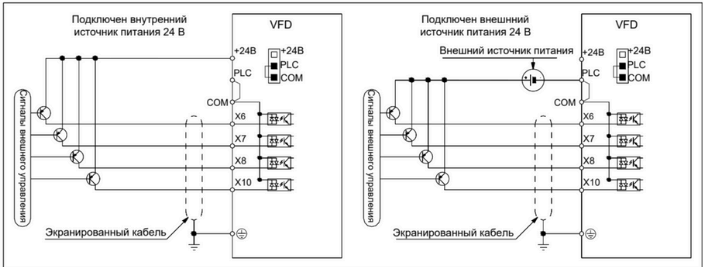
Рис. 2.1.1 Подключение PNP
