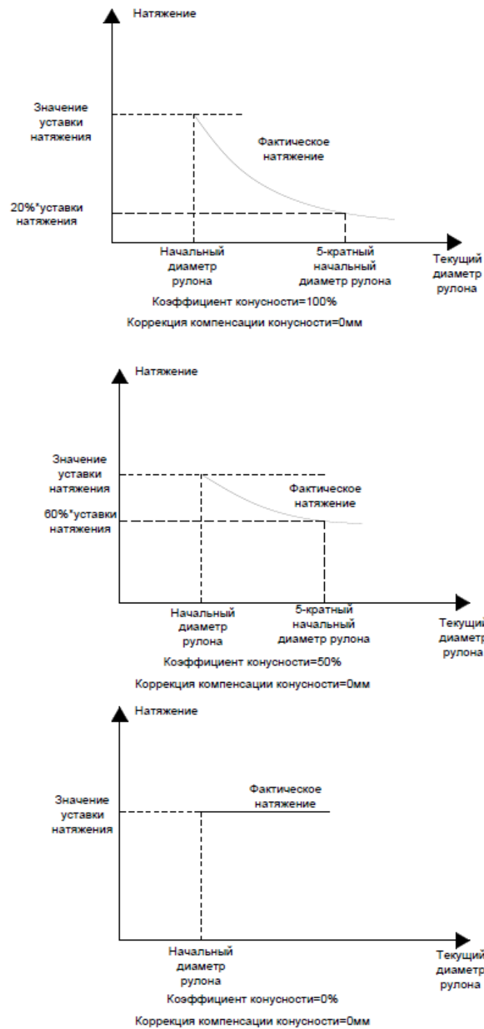
Рисунок 10.20-1 Изменение коэффициента конусности
