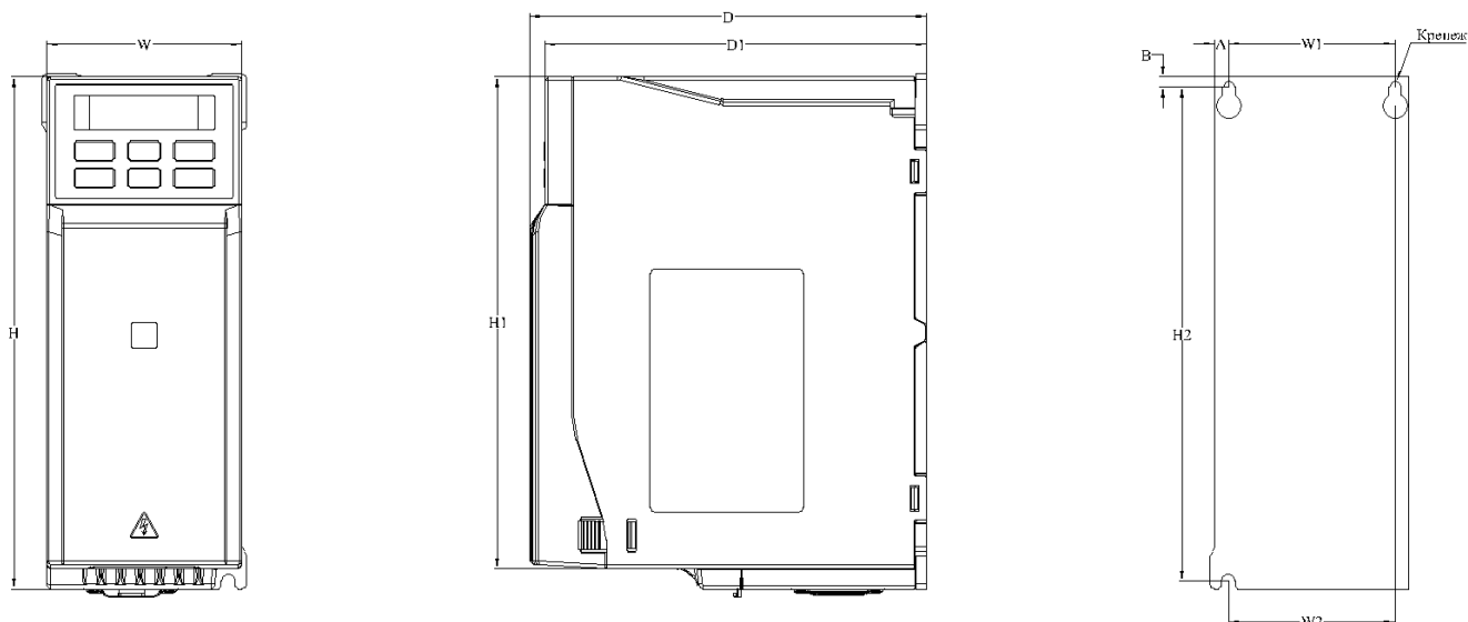
Рисунок 3.6—1 Чертеж преобразователя частоты типоразмер А01
