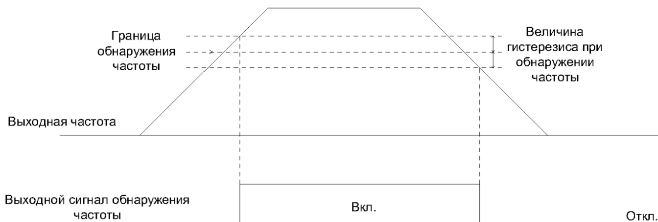
Рисунок 10.10-3 Определение частоты
