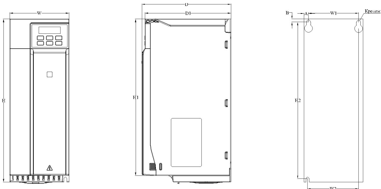
Рисунок 3.6-3 Чертеж преобразователя частоты типоразмер А03
