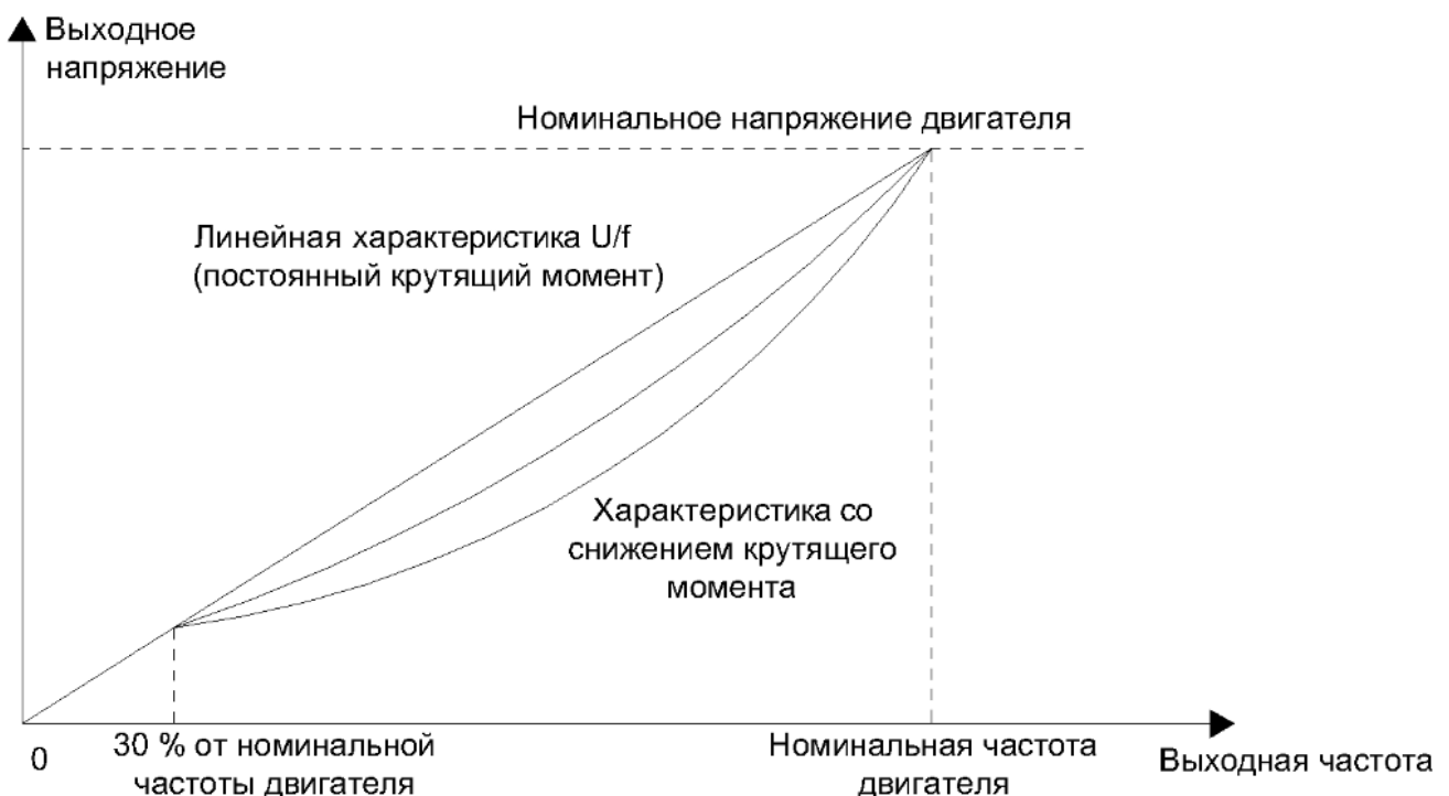
Рисунок 10.8-1 Усиление крутящего момента
