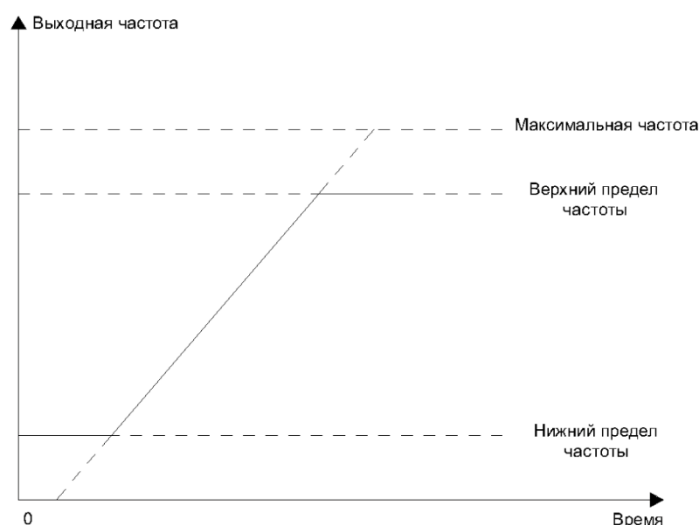
Рисунок 10.5-2 График, отображающий нижний и верхний пределы частот
