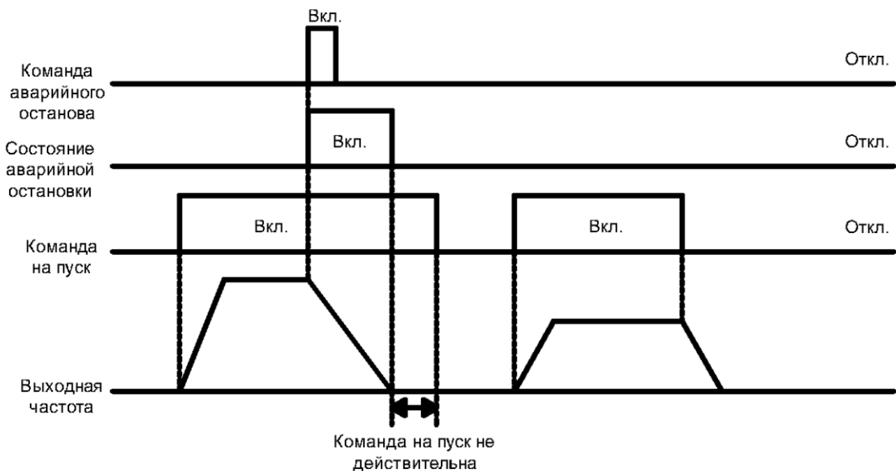
Рисунок 10.9-1 Диаграмма команды останова
