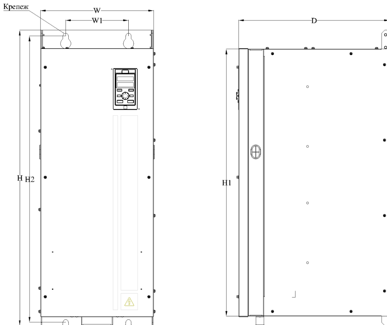
Рисунок 3.6-8 Чертеж преобразователя частоты типоразмер B03
