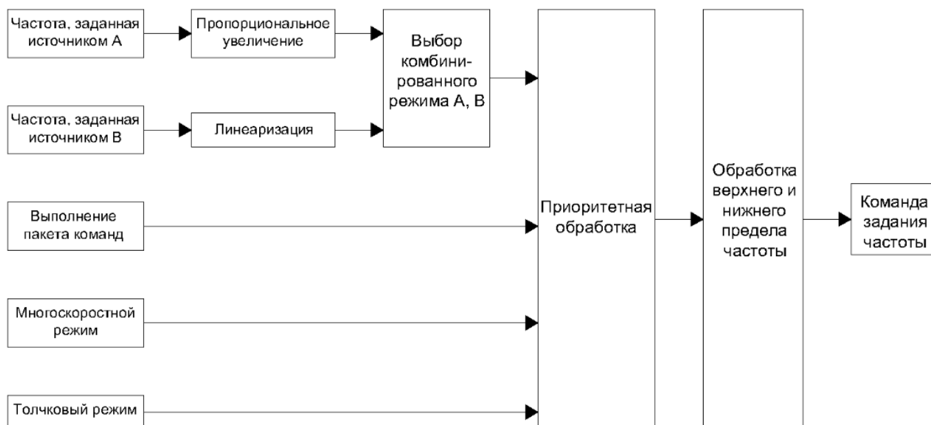
Рисунок 10.5-1 Схема задания частоты
