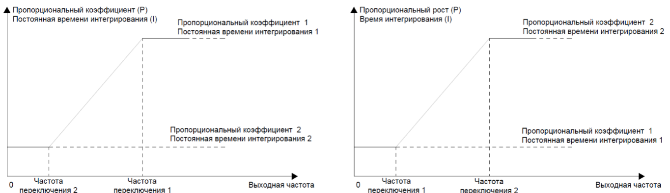
Рисунок 10.7-1 График настройки пропорционального коэффициента и постоянной времени интегрирования
