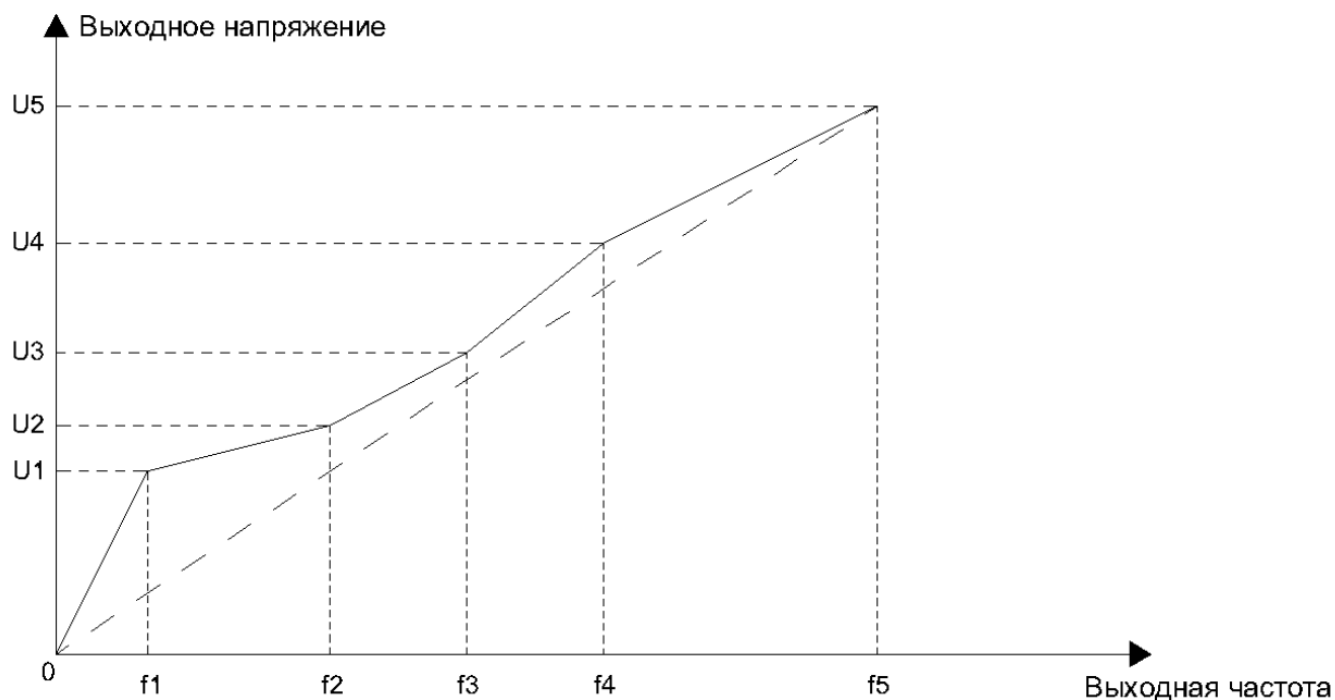
Рисунок 10.8-3 График пользовательской кривой
