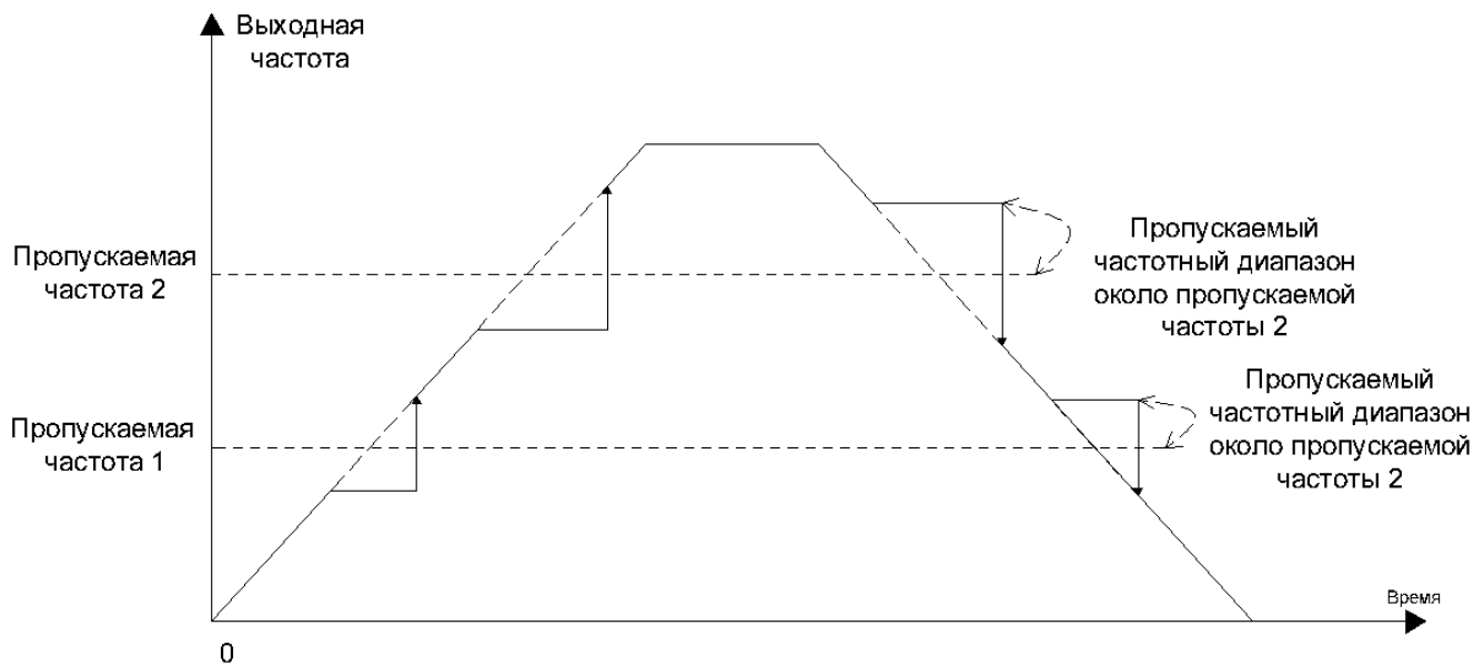
Рисунок 10.11-2 Кривые разгона/торможения с пропуском частот
