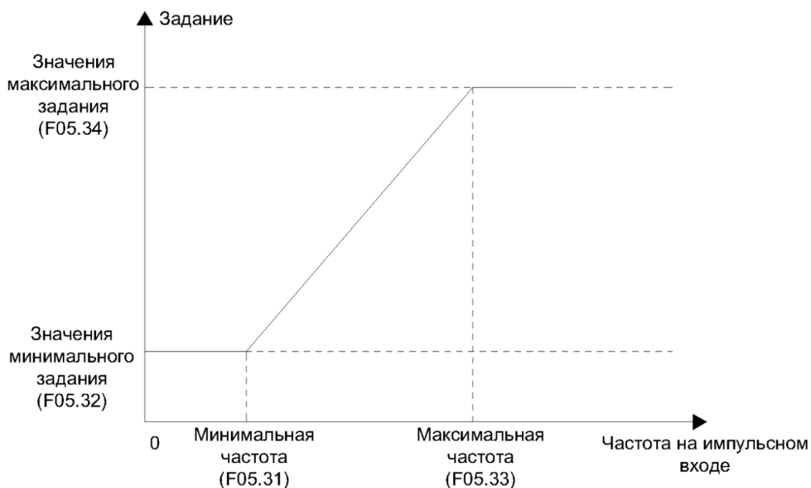
Рисунок 10.9-9 Обработка частоты сигнала, поступающего на импульсный вход
