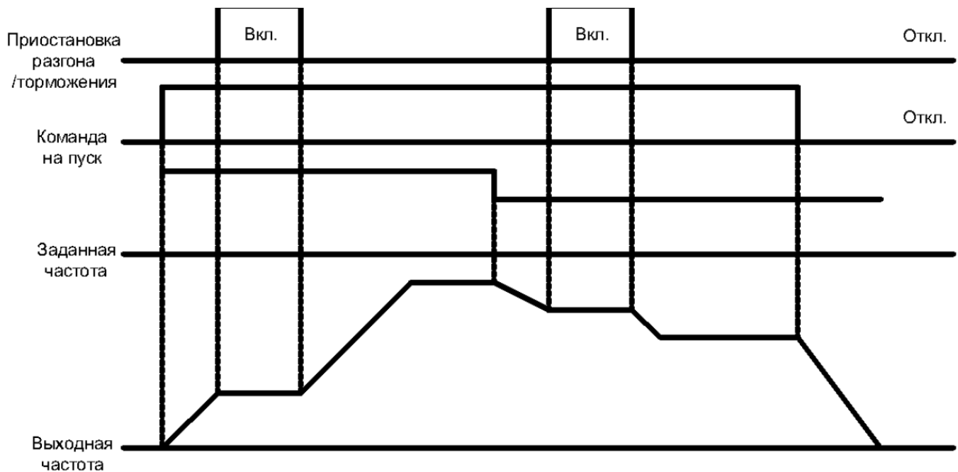
Рисунок 10.9-3 График приостановки разгона/торможения
