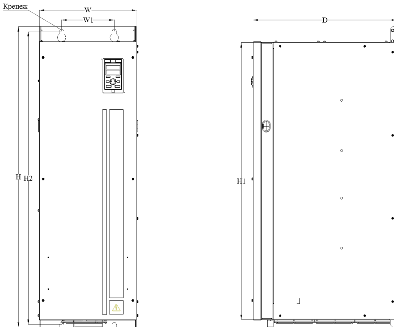
Рисунок 3.6-9 Чертеж преобразователя частоты типоразмер C01
