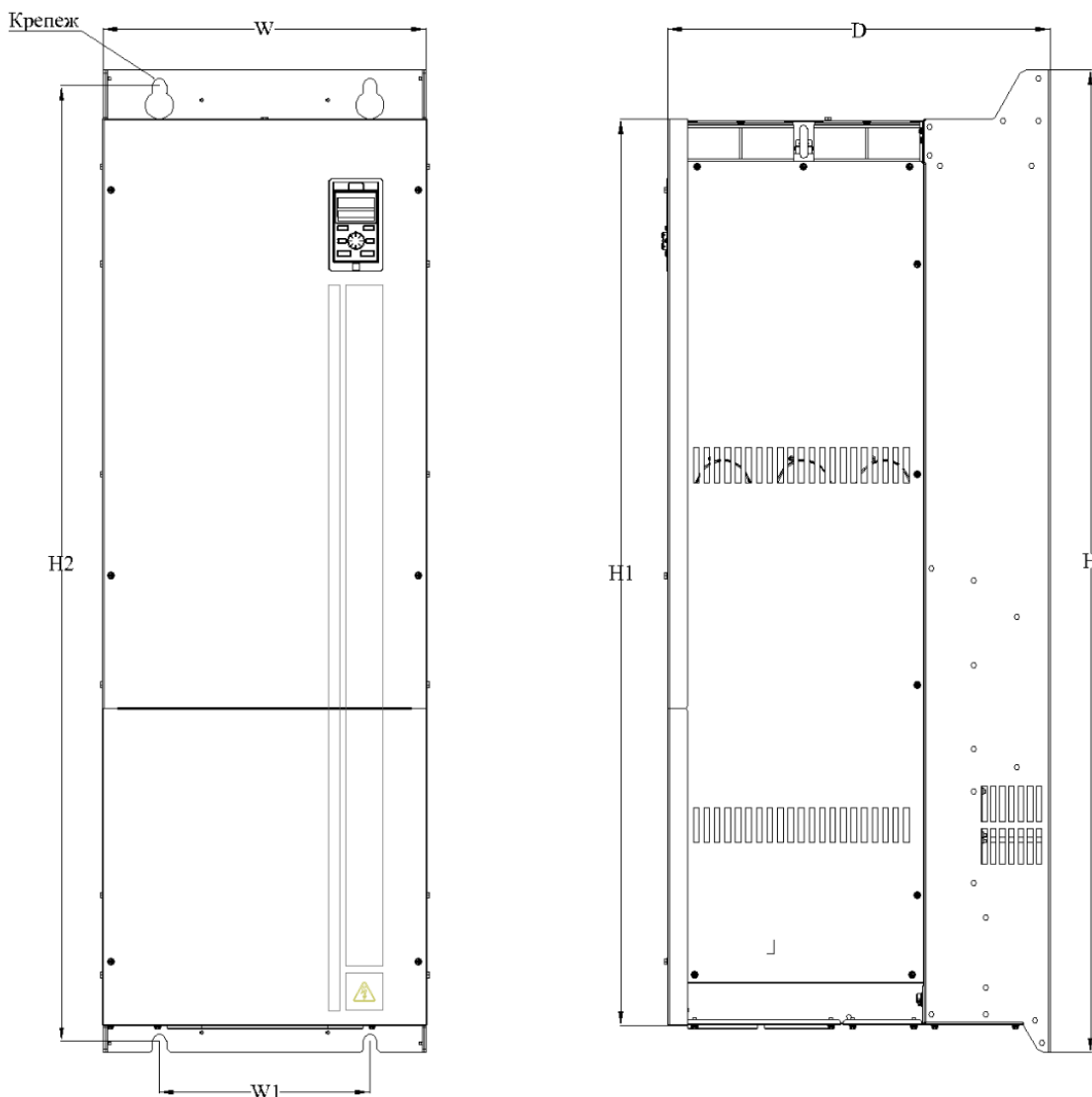
Рисунок 3.6-11 Чертеж преобразователя частоты типоразмер C03
