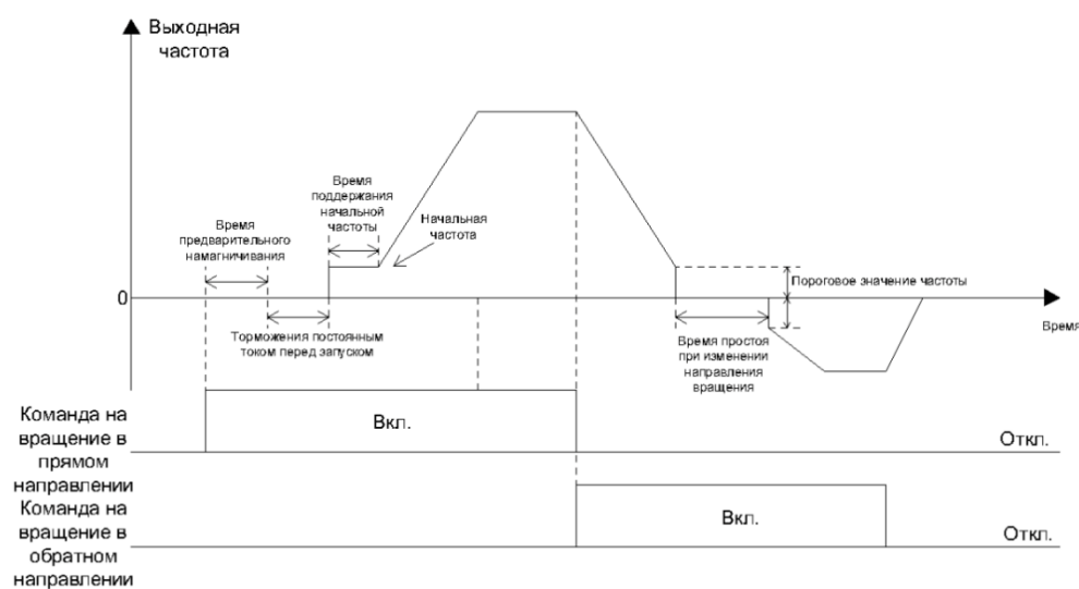
Рисунок 10.11-1 Кривые пуска, торможения и процесса переключения на реверсивный режим работы
