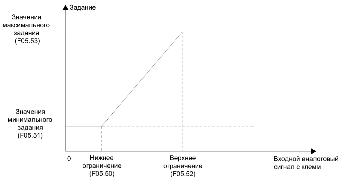
Рисунок 10.9-10 График линейной обработки аналогового сигнала
