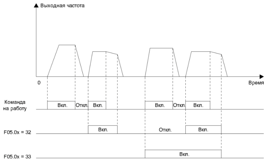
Рисунок 10.5-3 График времени разгона и торможения
