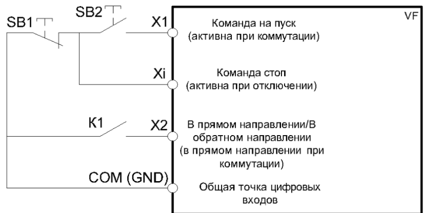
Рисунок 10.9-7 Трехпроводная схема управления 1
