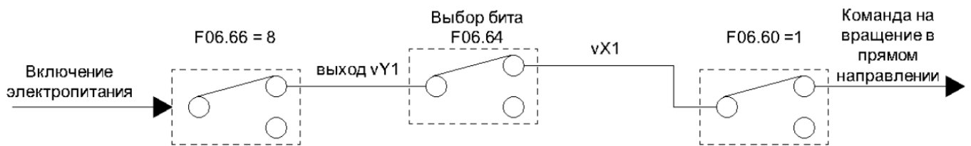
Рисунок 10.10-6 Схема автоматического запуска при включении питания
