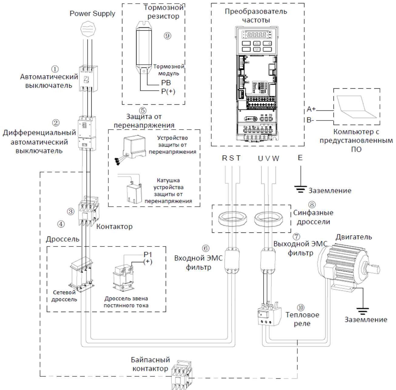
Рисунок 6.4-1 Подключение внешних устройств
