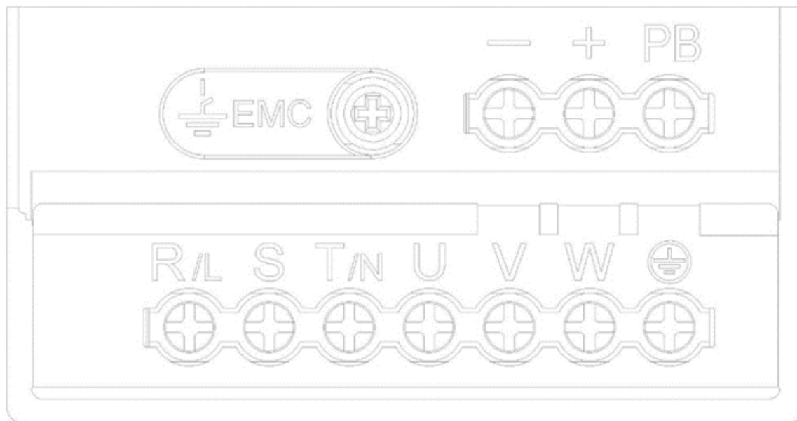
Рисунок 4.4-2 Расположение клемм
