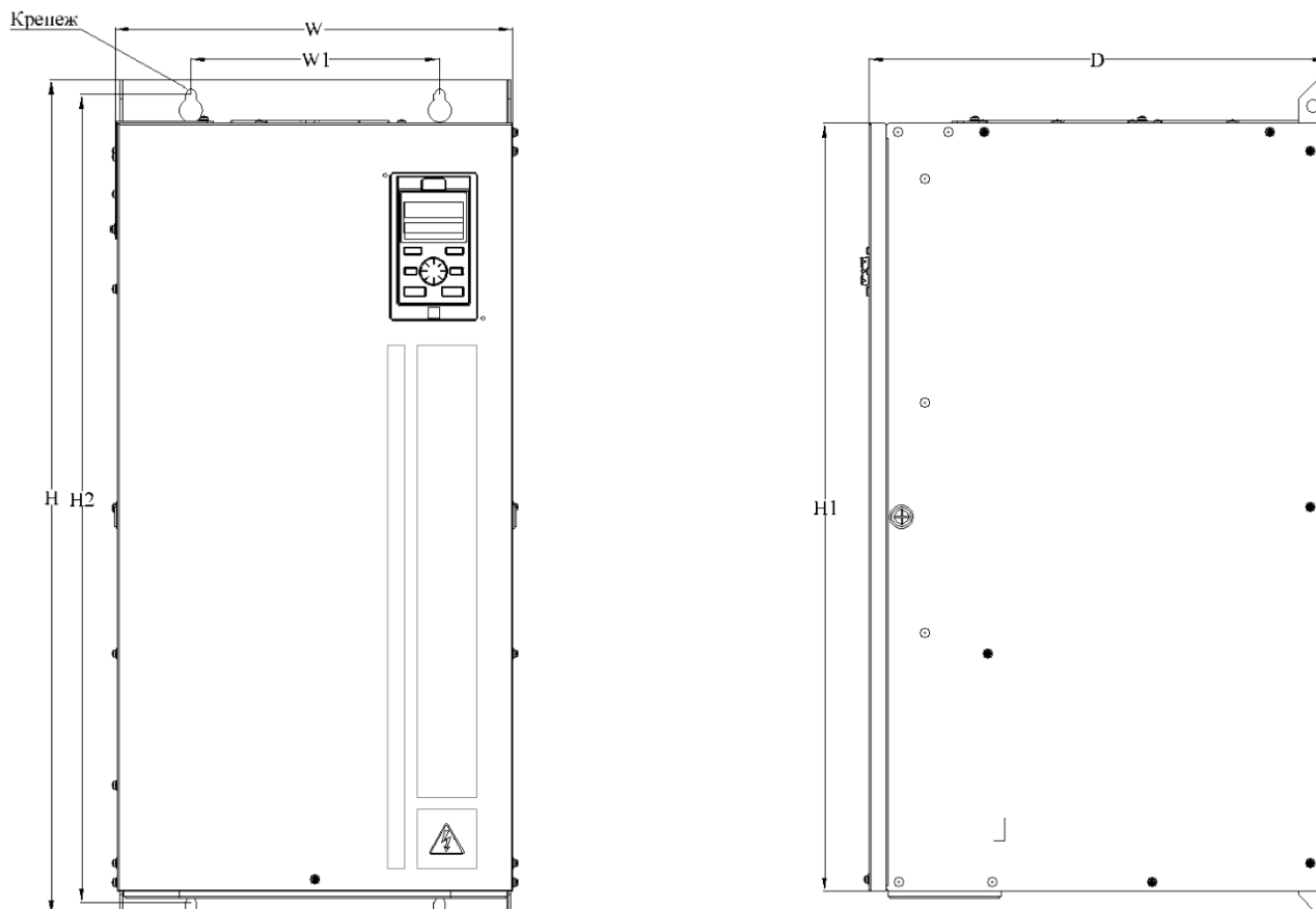
Рисунок 3.6-7 Чертеж преобразователя частоты типоразмер B02
