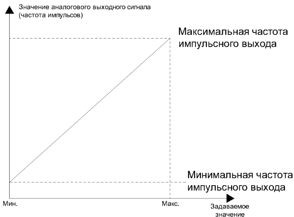
Рисунок 10.10-2 График частоты сигнала аналогового выхода
