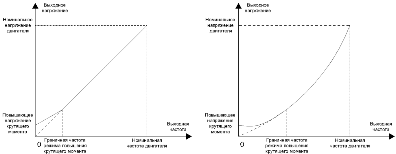
Рисунок 10.8-2 Графики изменения характеристики для линейной и квадратичной кривой
