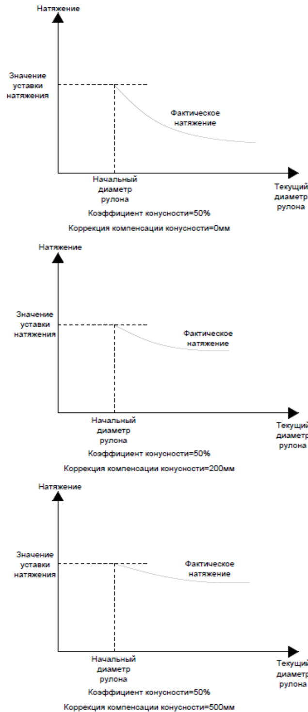
Рисунок 10.20-2 Изменение коррекции компенсации конусности
