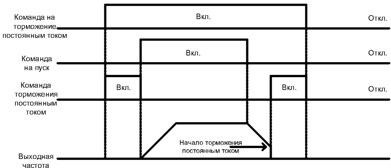
Рисунок 10.9-4 График торможения постоянным током
