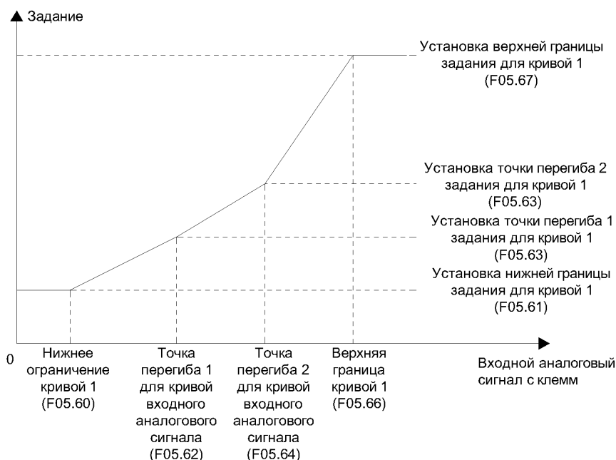
Рисунок 10.9-11 Кривая 1 входного аналогового сигнала
