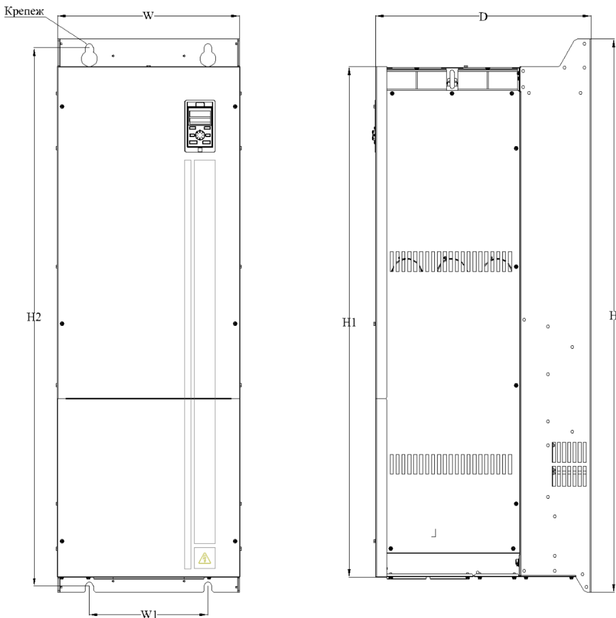
Рисунок 3.6-12 Чертеж преобразователя частоты типоразмер C04
