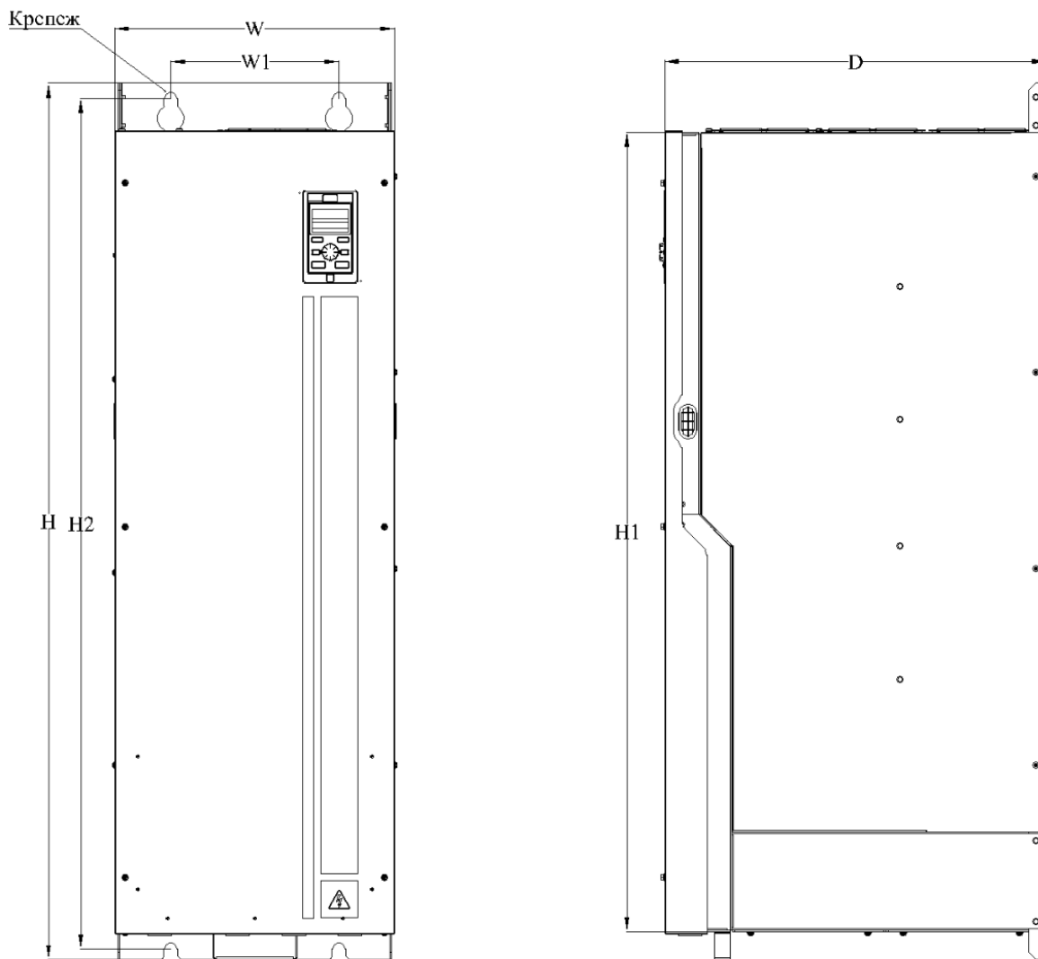
Рисунок 3.6-10 Чертеж преобразователя частоты типоразмер C02
