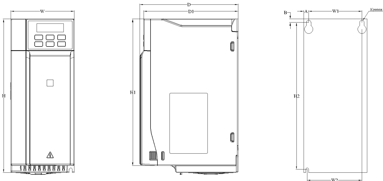
Рисунок 3.6-2 Чертеж преобразователя частоты типоразмер A02
