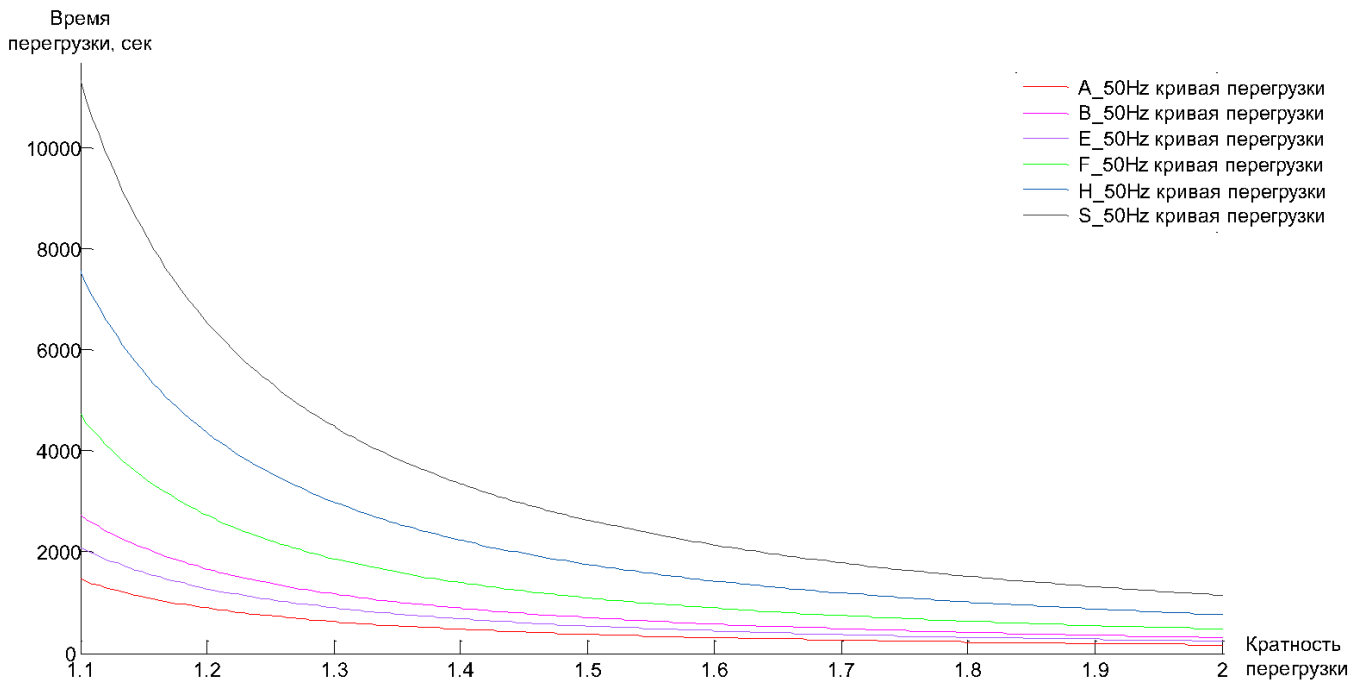
Рисунок 10.14-1 График перегрузки для разных классов изоляции электродвигателя при 50 Гц
