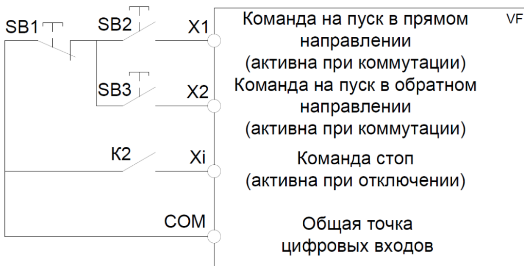
Рисунок 10.9-8 Трехпроводная схема управления 2
