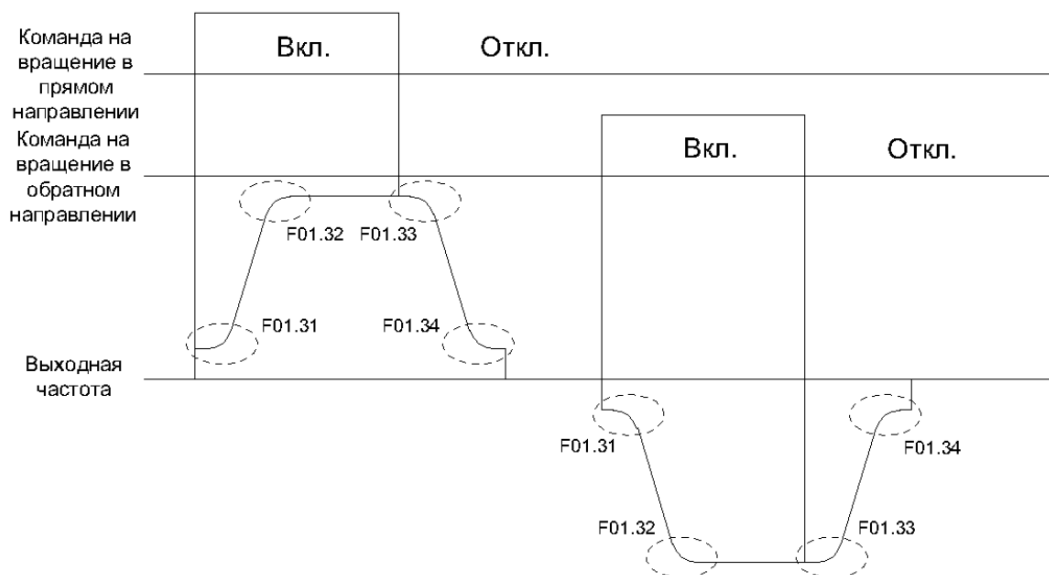
Рисунок 10.5-5 График кривой S
