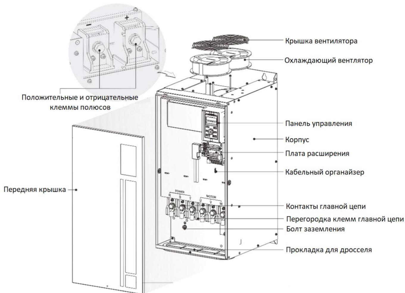
Рисунок 4.4-1 Конструкция преобразователя частоты с металлическим корпусом серии TG910
