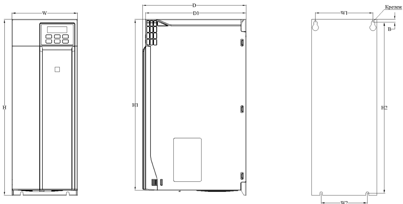
Рисунок 3.6-4 Чертеж преобразователя частоты типоразмер А04
