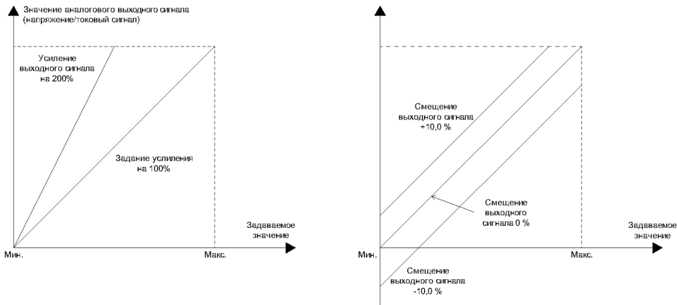
Рисунок 10.10-1 График усиления и смещения аналогового сигнала
