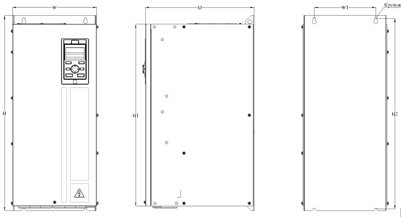
Рисунок 3.6-6 Чертеж преобразователя частоты типоразмер B01
