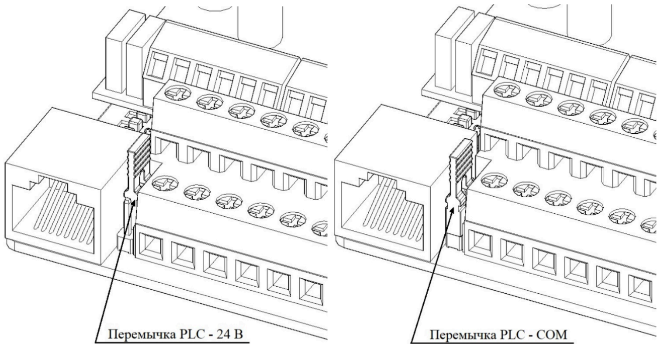
Рисунок 4.7-3 Схема подключения перемычек «+24В», «PLC», «COM»
