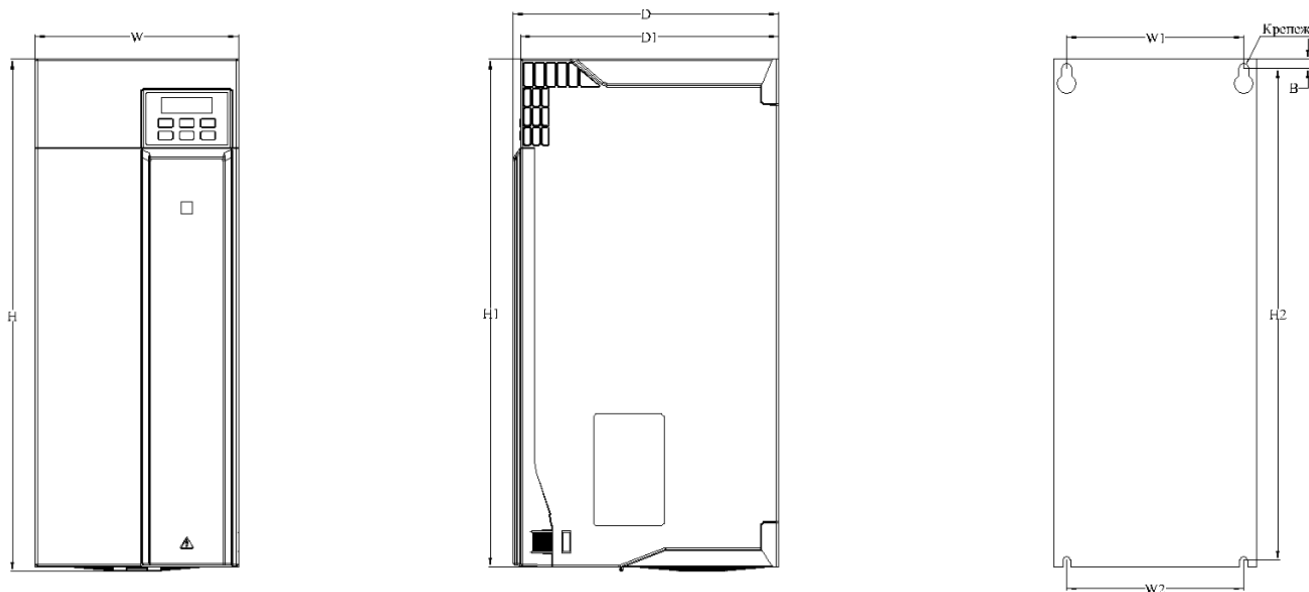
Рисунок 3.6-5 Чертеж преобразователя частоты типоразмер А05
