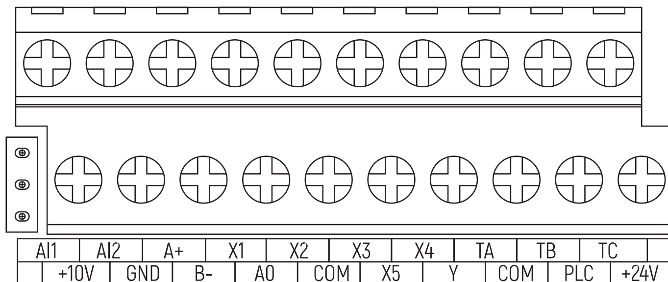
Рисунок 4.5-2 Расположение клемм цепи управления
