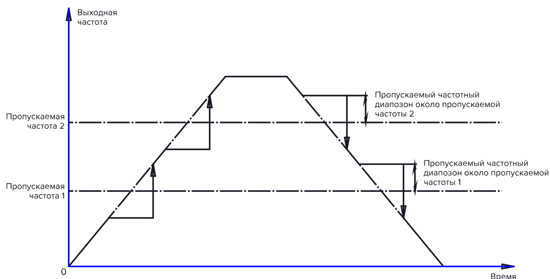
Рисунок 10.11-2 Кривые разгона/торможения с пропуском частот
