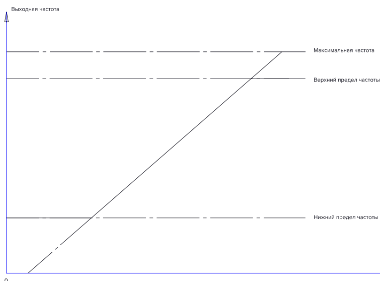
Рисунок 10.5-2 График, отображающий нижний и верхний пределы частот
