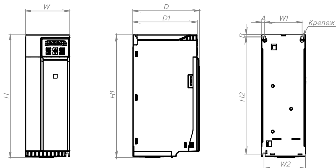
Рисунок 3.6-3 Чертеж преобразователя частоты типоразмер A03
