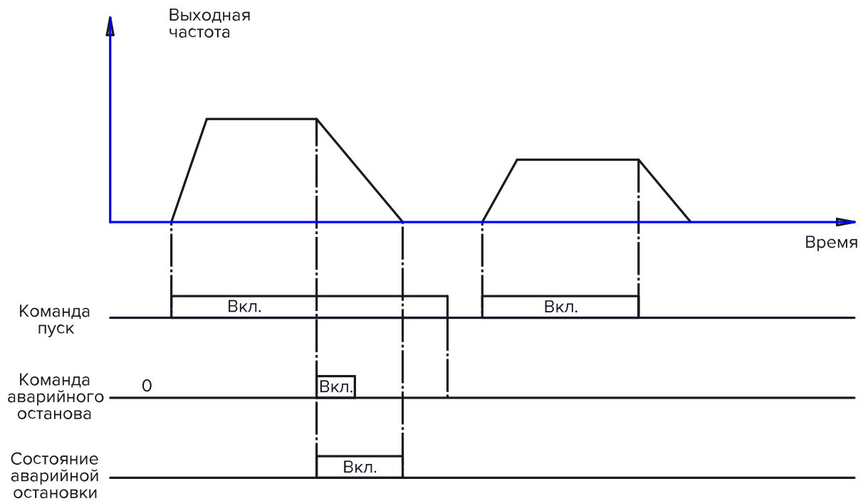
Рисунок 10.9-1 Диаграмма команды останова
