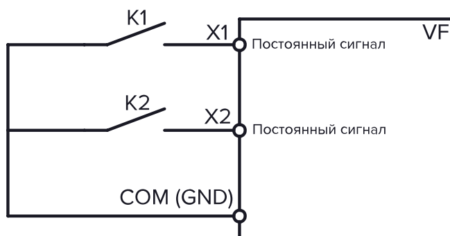
Рисунок 10.9-5 Двухпроводная схема управления 1
