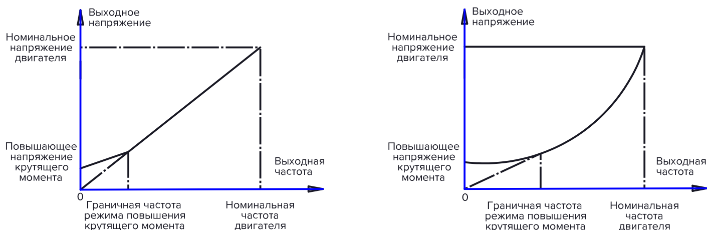
Рисунок 10.8-2 Графики изменения характеристики для линейной и квадратичной кривой
