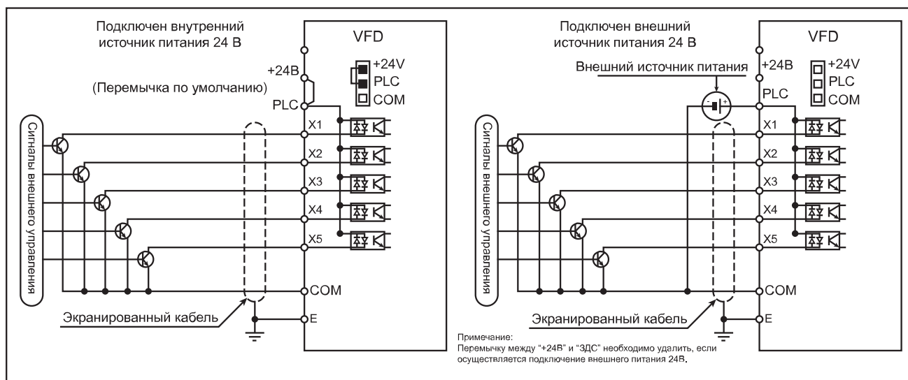
Рисунок 4.7-2 Способ подключения логики NPN
