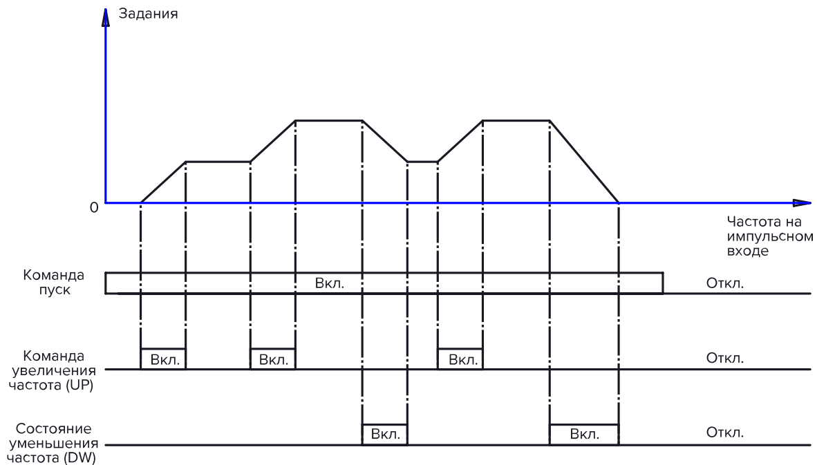
Рисунок 10.9-2 График частоты с применением функций увеличения и уменьшения
