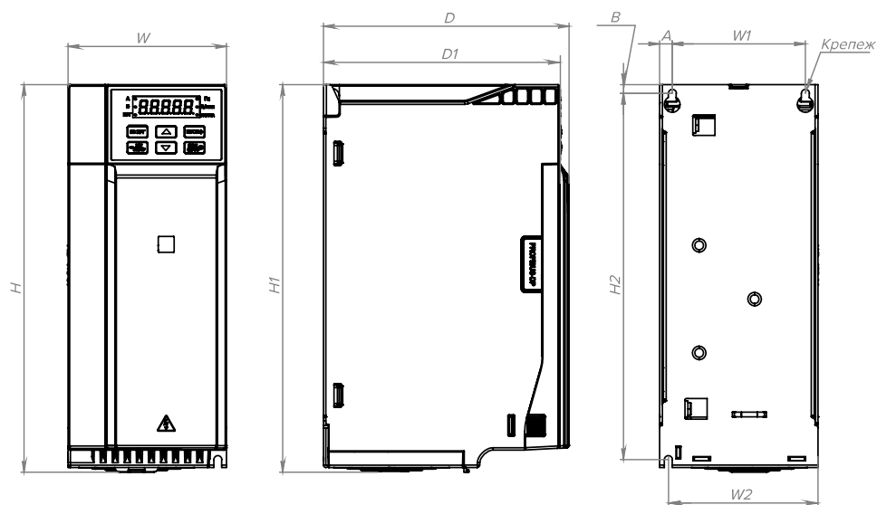
Рисунок 3.6-2 Чертеж преобразователя частоты типоразмер A02
