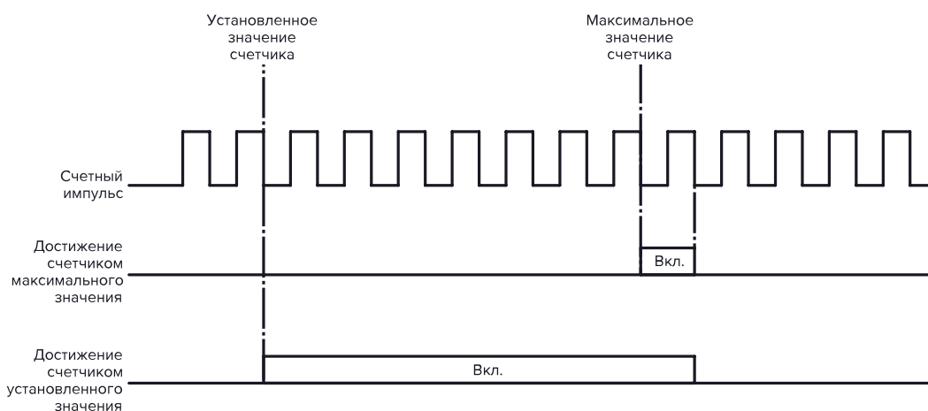
Рисунок 10.12-1 Изменение значения счетчика при достижении максимального и установленного значений
