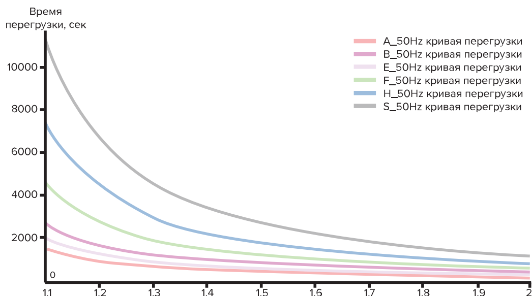
Рисунок 10.14-1 График перегрузки для разных классов изоляции электродвигателя при 50 Гц
