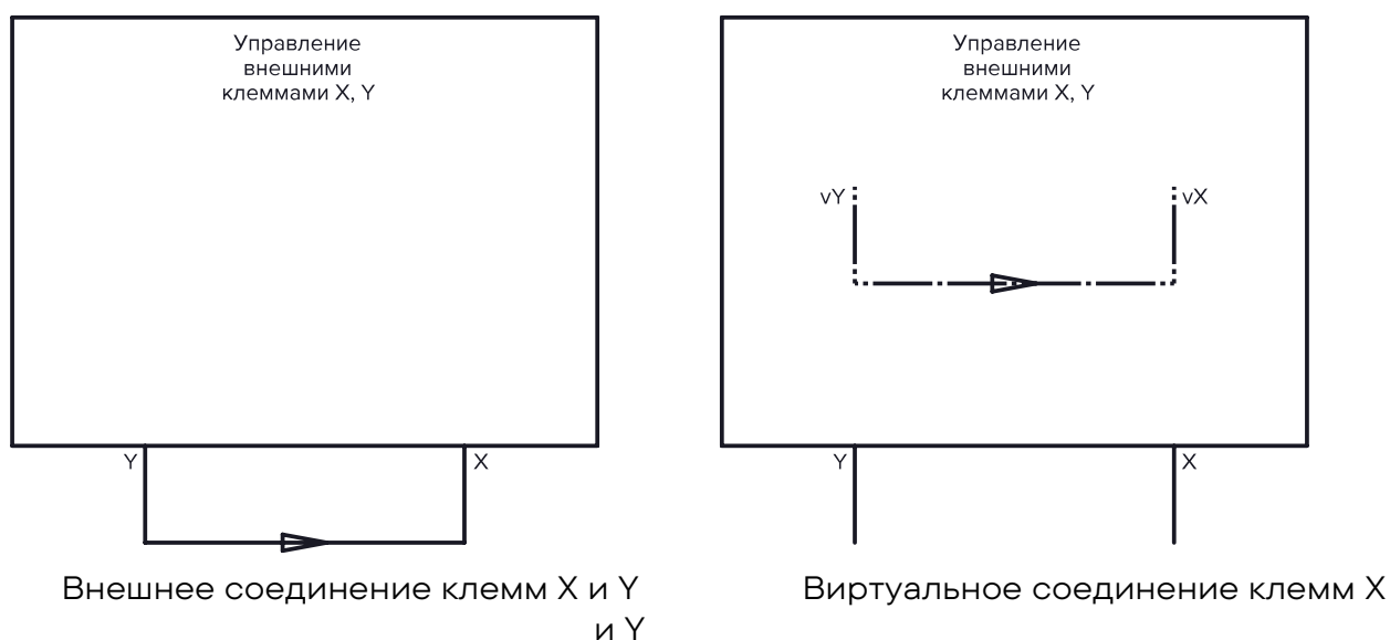
Рисунок 10.10–5 Работа функции виртуальных клемм X и Y
