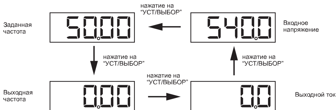
Рисунок 5.5-2 Переключение контролируемых параметров
