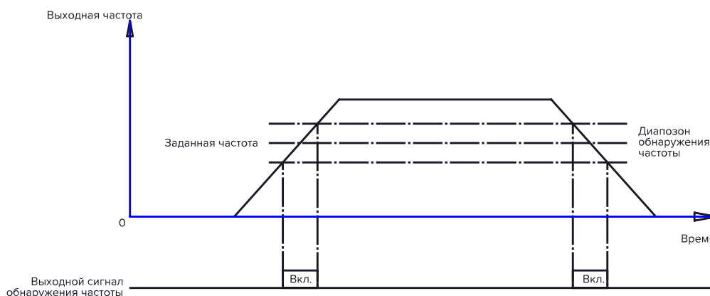
Рисунок 10.10-4 График выходного сигнала, когда частота входит в диапазон обнаружения
