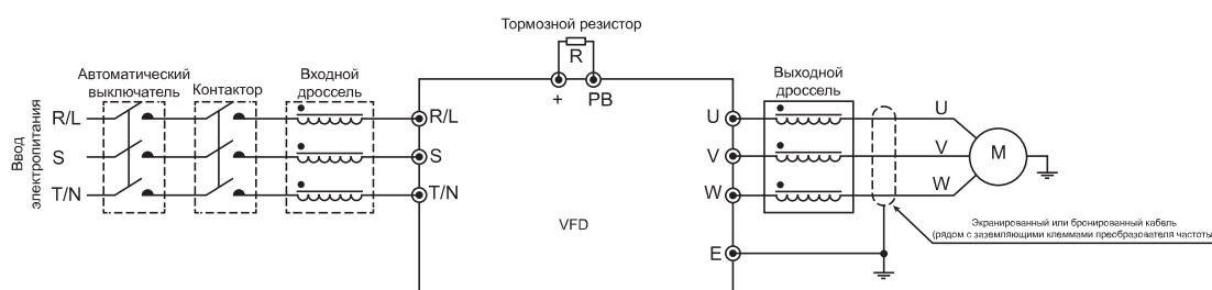
Рисунок 4.4-1 Типовая схема подключения преобразователя частоты
