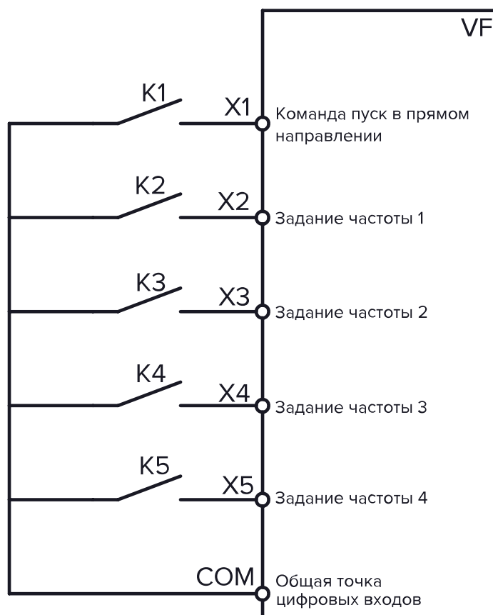
Рисунок 10.18-1 Схема подключения клемм
