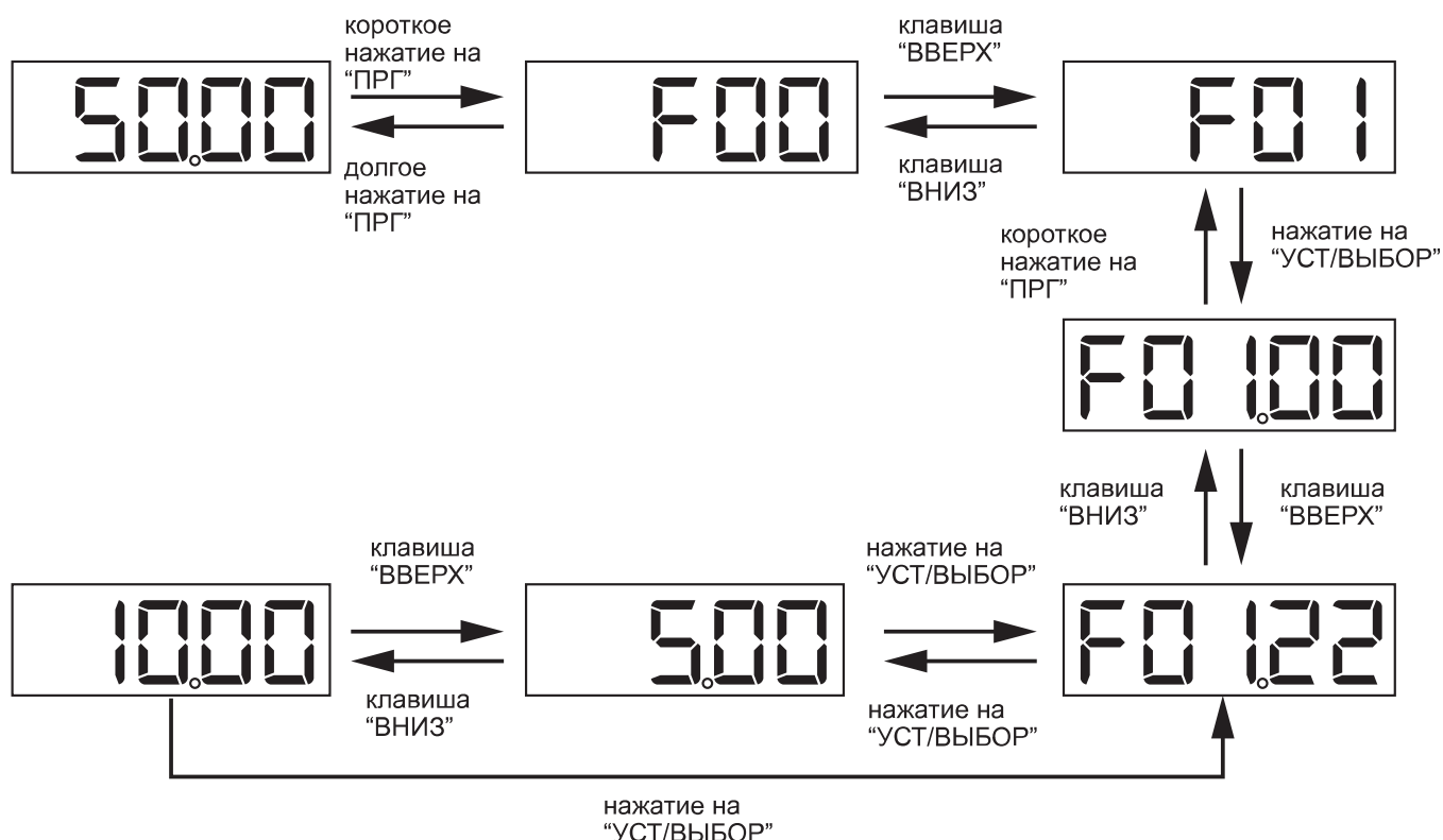
Рисунок 5.5-1 Базовые операции на панели управления
