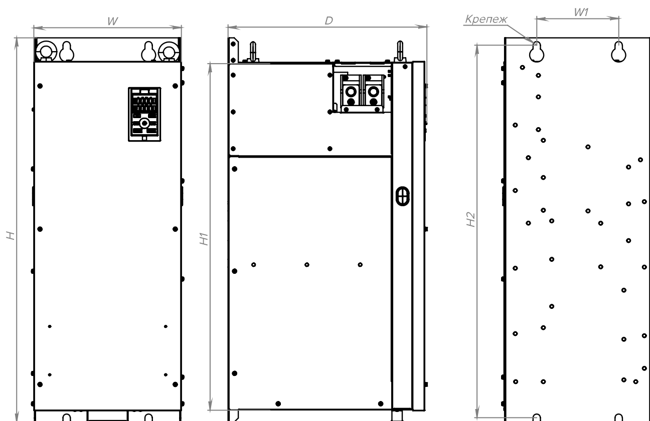
Рисунок 3.6-12 Чертеж преобразователя частоты типоразмер C04
