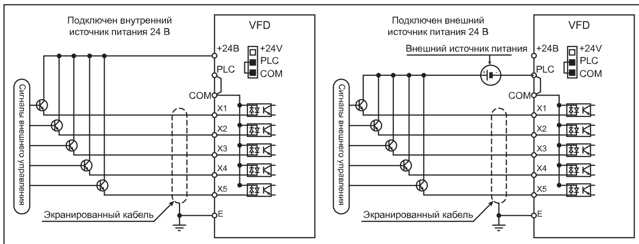
Рисунок 4.7-1 Способ подключения логики PNP
