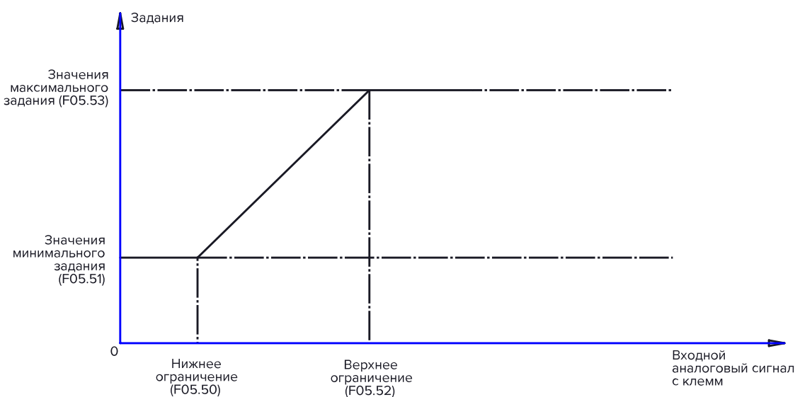
Рисунок 10.9-10 График линейной обработки аналогового сигнала
