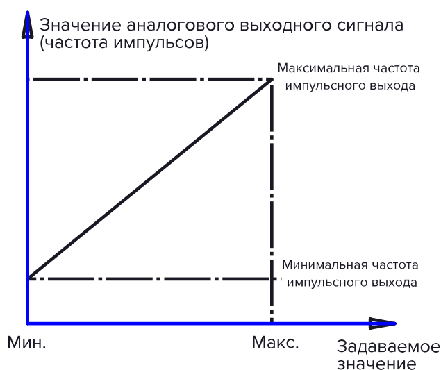
Рисунок 10.10-2 График частоты сигнала аналогового выхода
