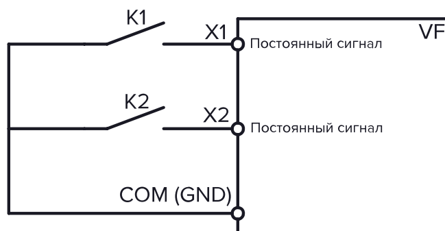
Рисунок 10.9-6 Двухпроводная схема управления 2
