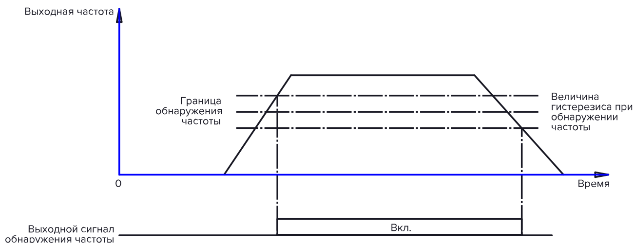
Рисунок 10.10-3 Определение частоты
