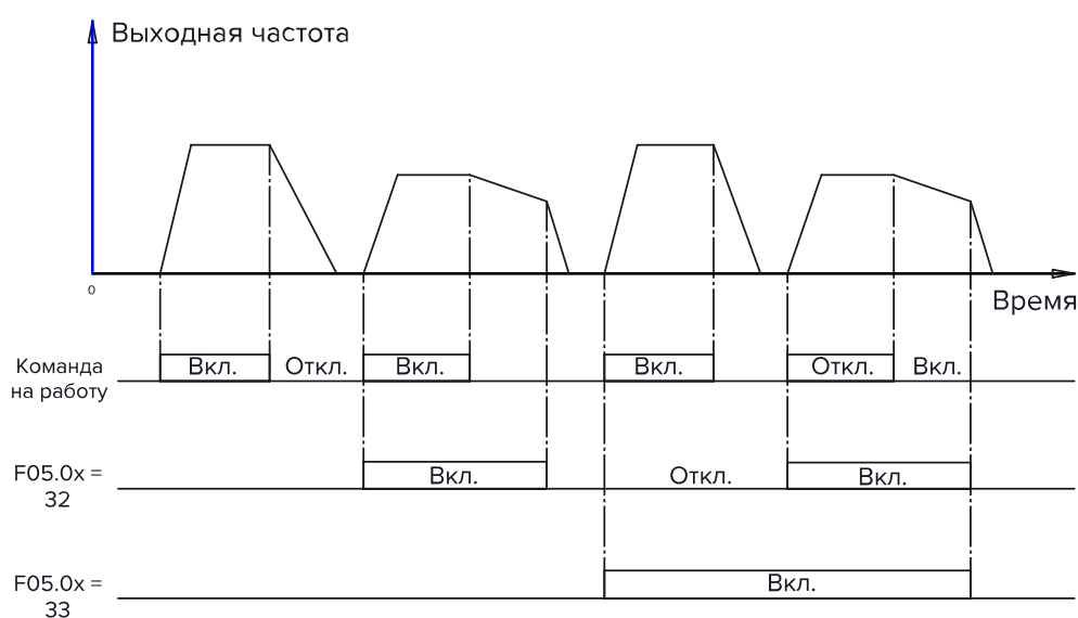
Рисунок 10.5-3 График времени разгона и торможения
