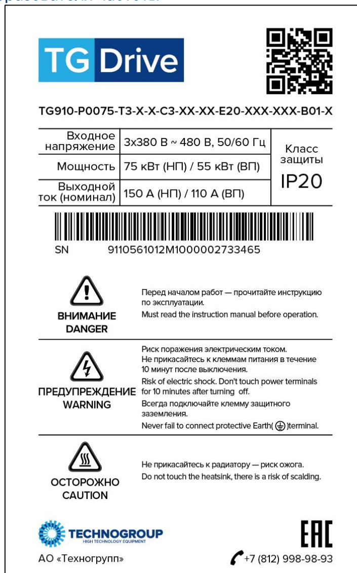
Рисунок 1.3—1 Пример маркировки преобразователя частоты
