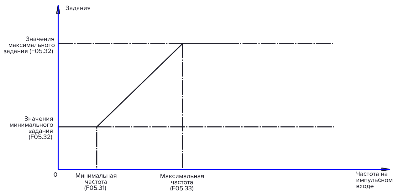
Рисунок 10.9-9 Обработка частоты сигнала, поступающего на импульсный вход
