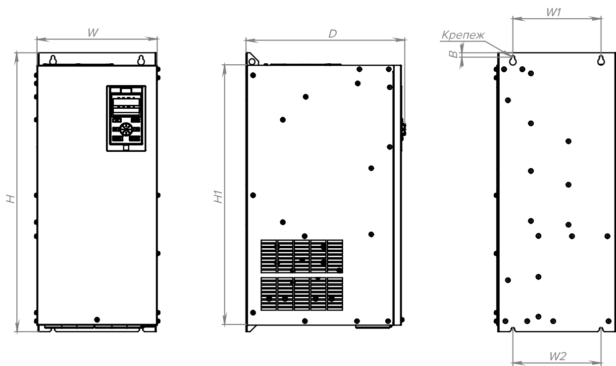
Рисунок 3.6-6 Чертеж преобразователя частоты типоразмер B01
