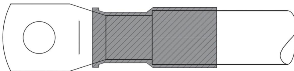
Рис. 4.10-4 Пример применения термоизоляционной трубки (выделена штриховкой) для изоляции соединения кабельного наконечника и силового кабеля
