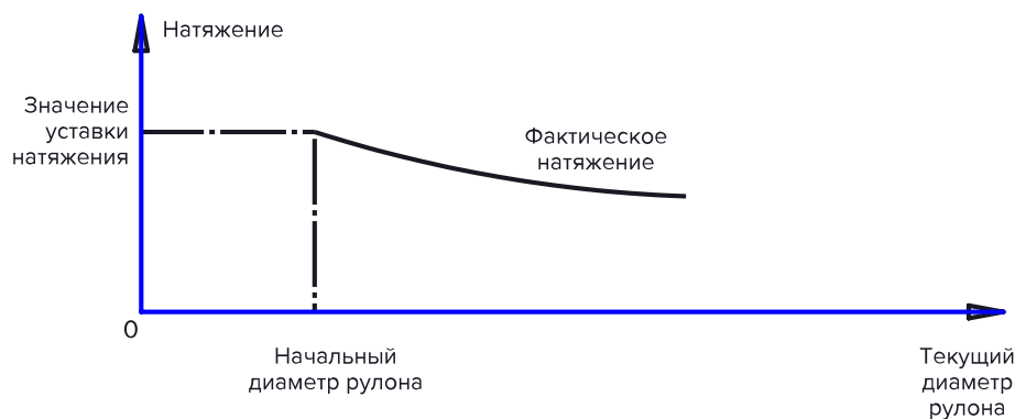
Рисунок 10.20-2 Изменение коррекции компенсации конусности
