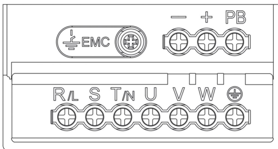
Рисунок 4.4-3 Расположение клемм
