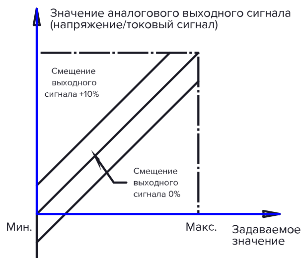
Рисунок 10.10-1 График усиления и смещения аналогового сигнала
