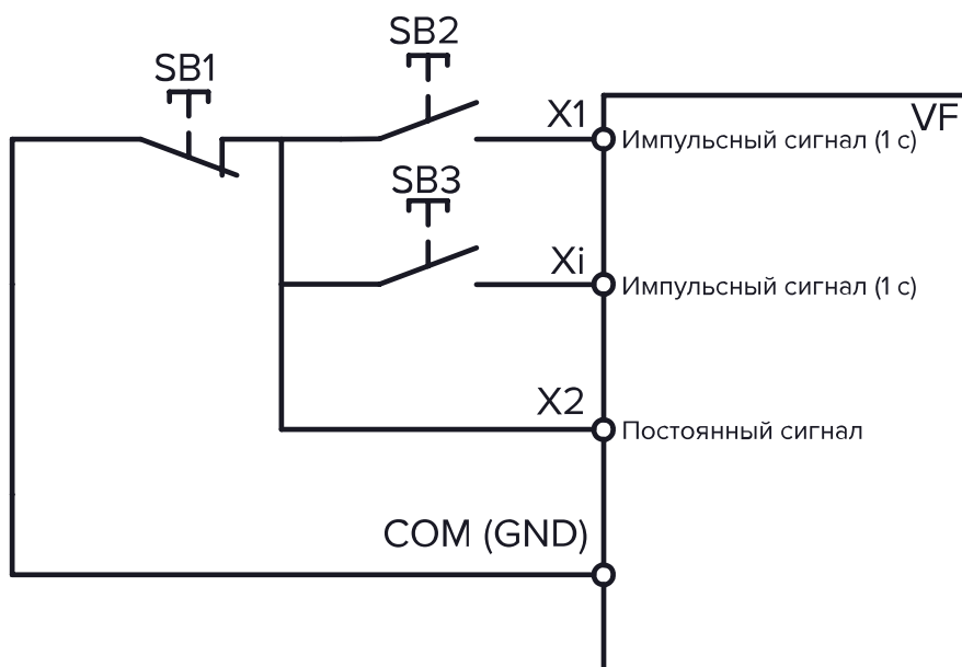
Рисунок 10.9–8 Трёхпроводная схема управления 2
