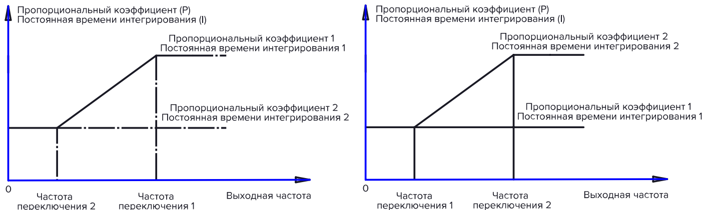
Рисунок 10.7-1 График настройки пропорционального коэффициента и постоянной времени интегрирования
