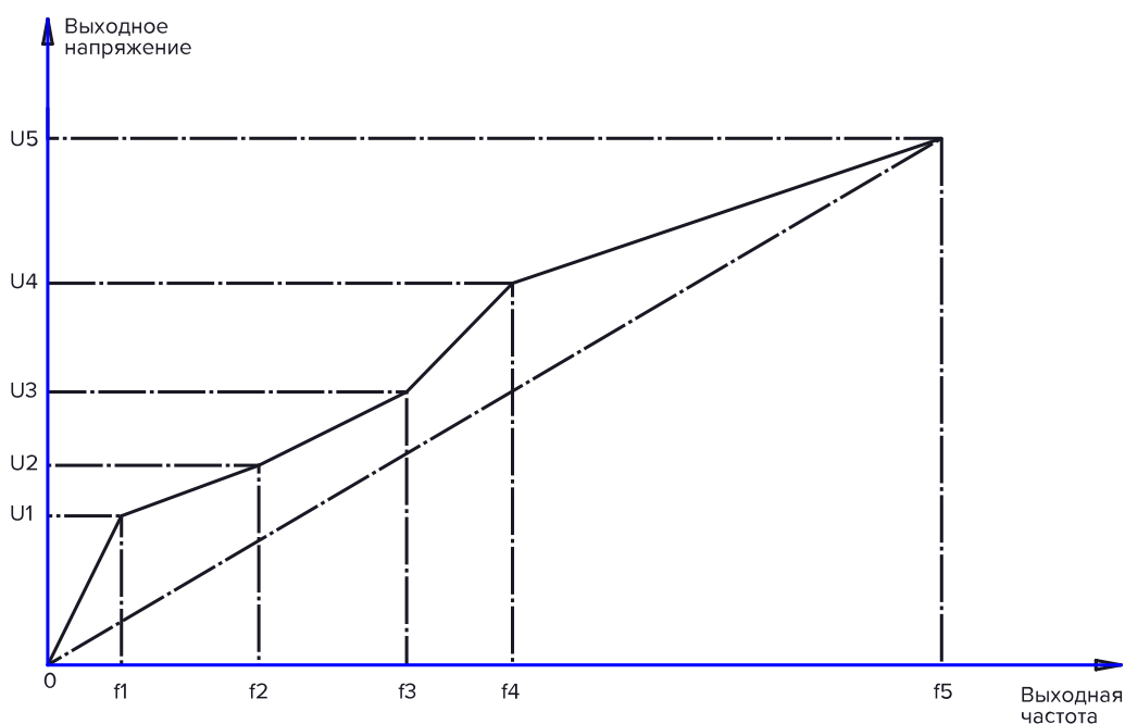
Рисунок 10.8-3 График пользовательской кривой
