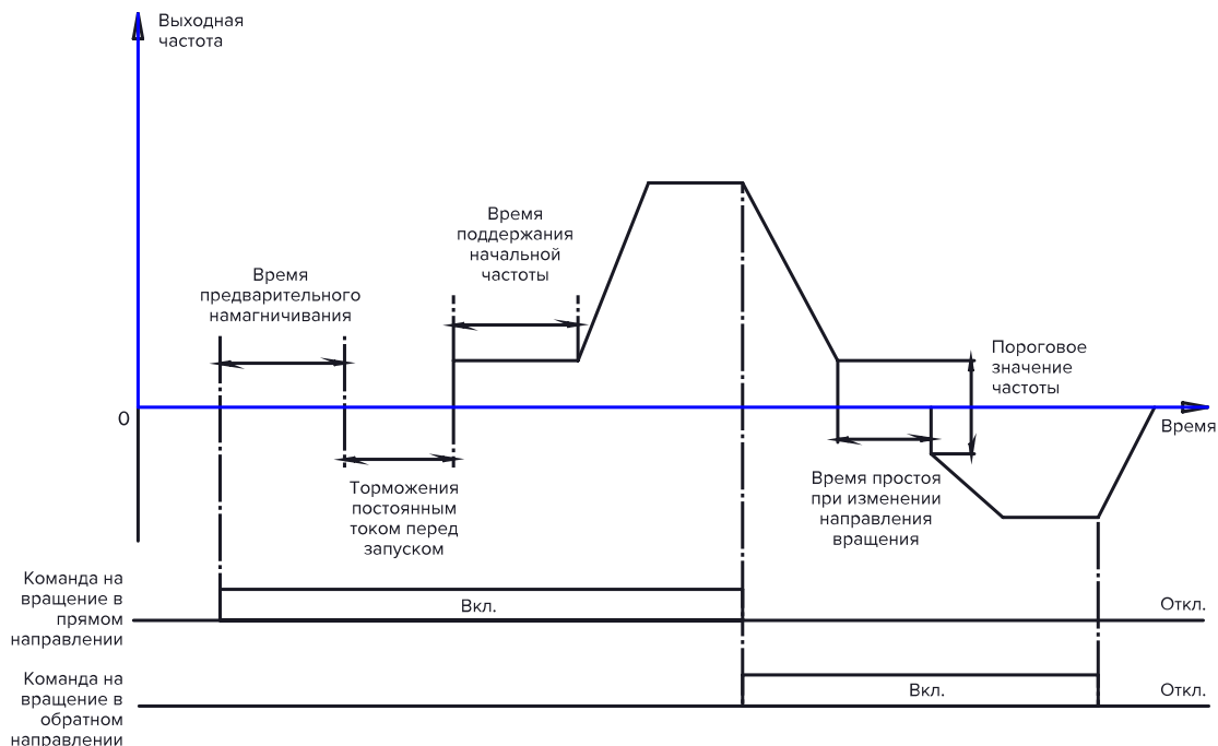
Рисунок 10.11-1 Кривые пуска, торможения и процесса переключения на реверсивный режим работы
