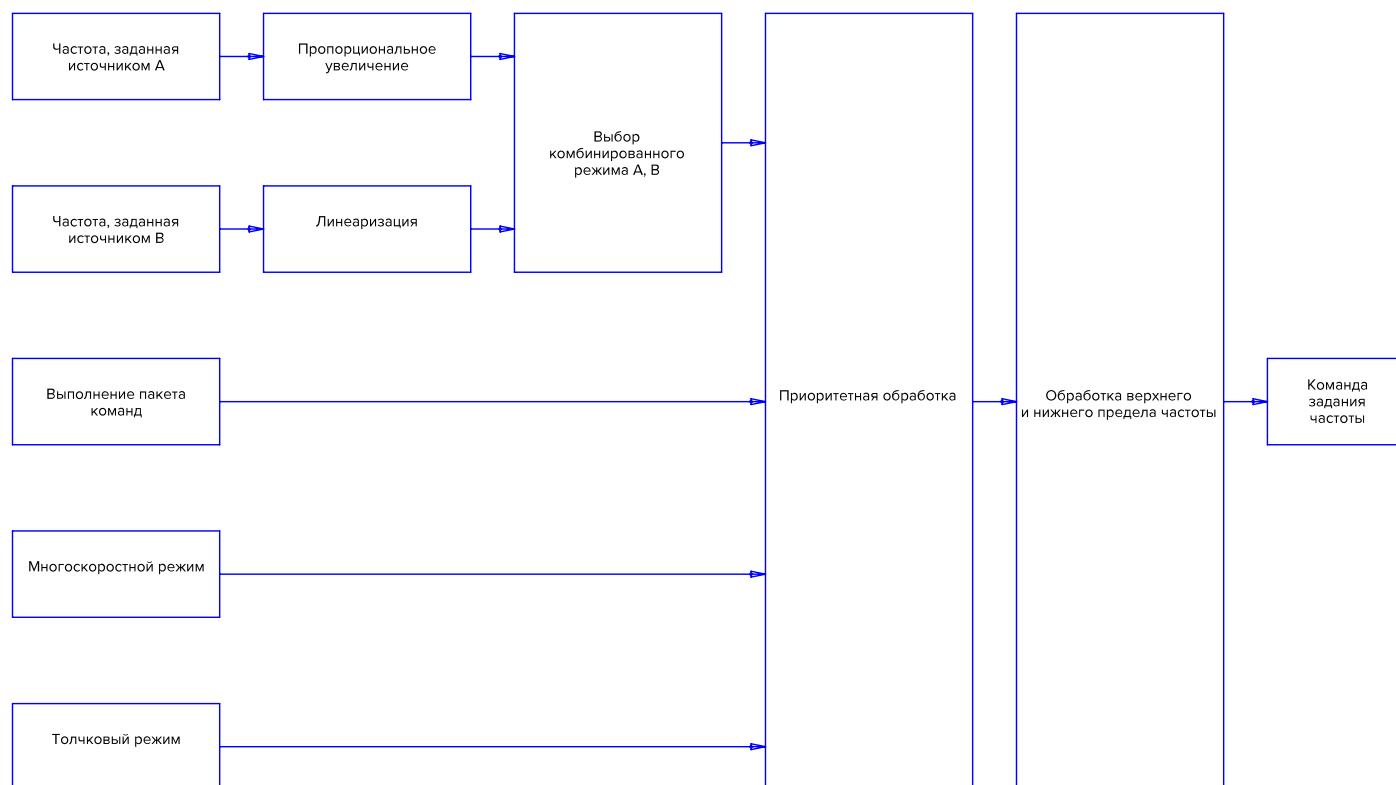
Рисунок 10.5–1 Схема задания частоты
