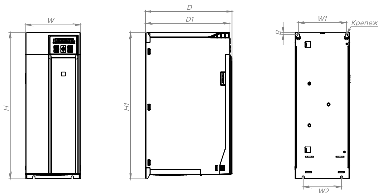
Рисунок 3.6-5 Чертеж преобразователя частоты типоразмер A05
