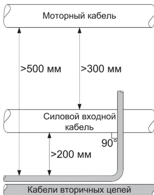
Рис. 4.10-5 Принцип прокладки силовых и управляющих кабелей
