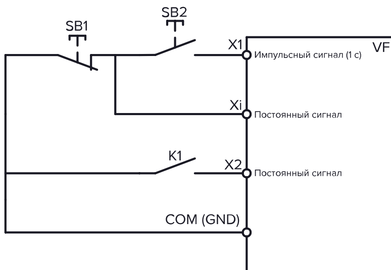
Рисунок 10.9-7 Трехпроводная схема управления 1
