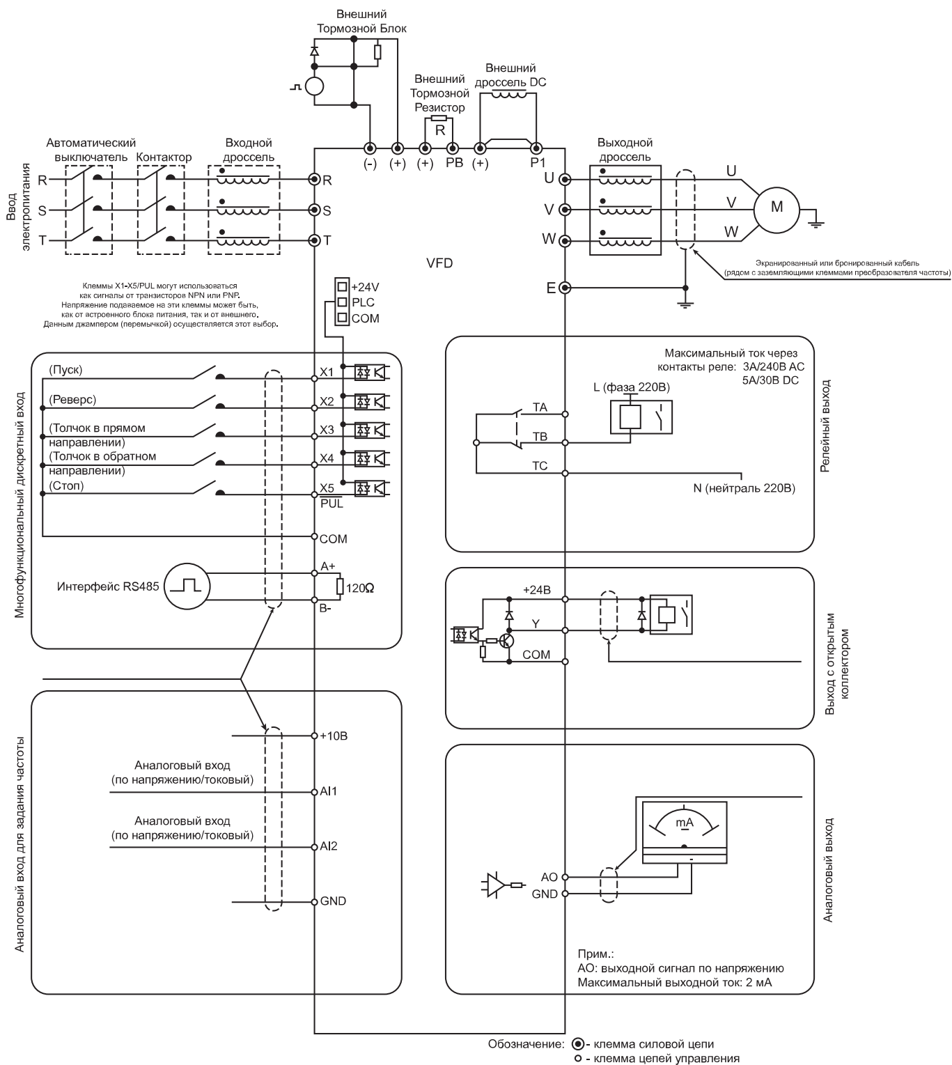
Рисунок 4.5-1 Схема внешних подключений
