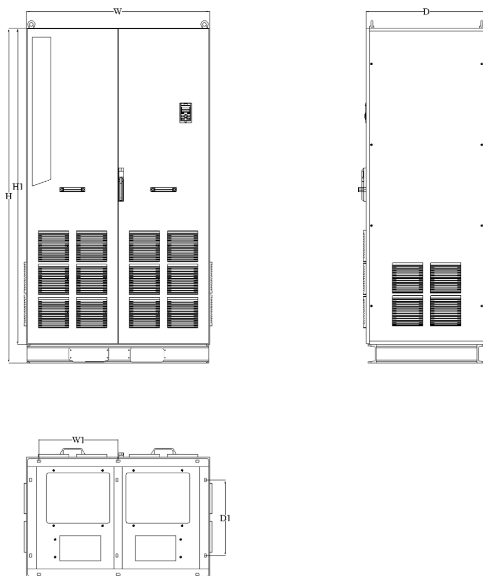
Рисунок 3.6-13 Чертеж преобразователя частоты типоразмер D01
