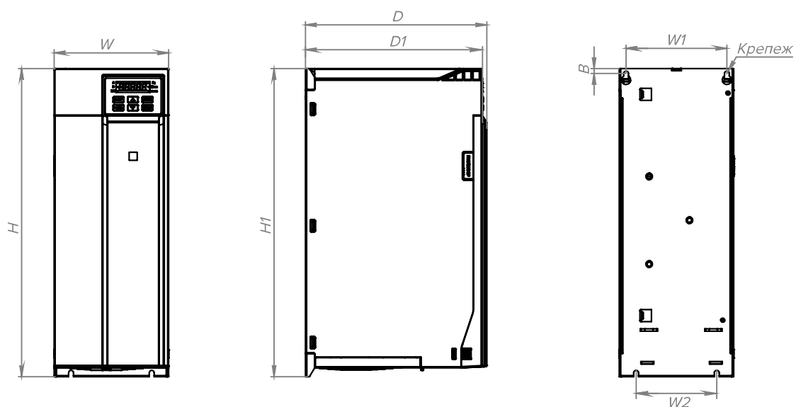
Рисунок 3.6-4 Чертеж преобразователя частоты типоразмер A04
