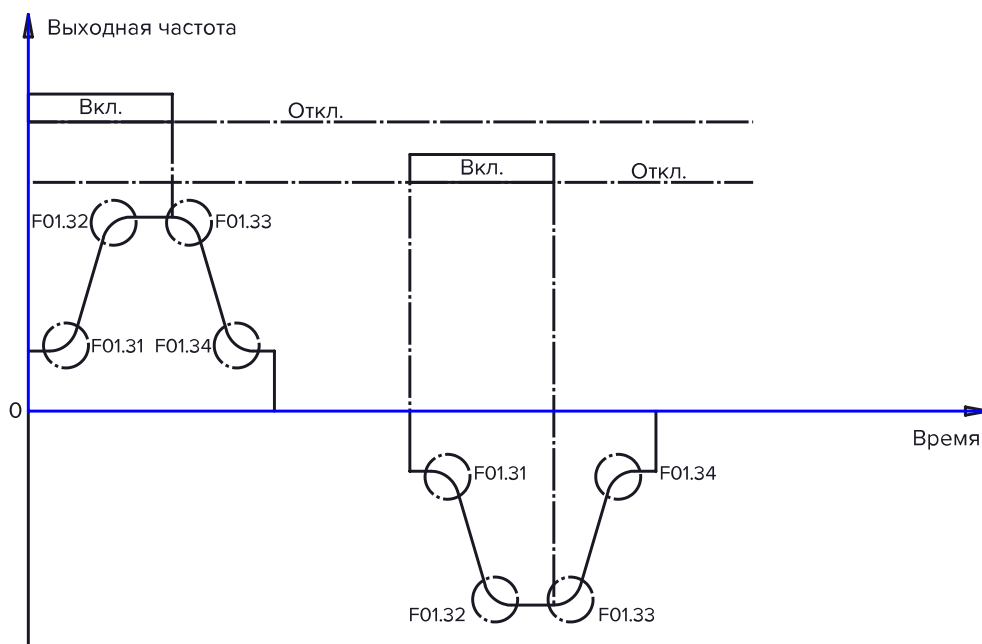
Рисунок 10.5-5 График кривой S
