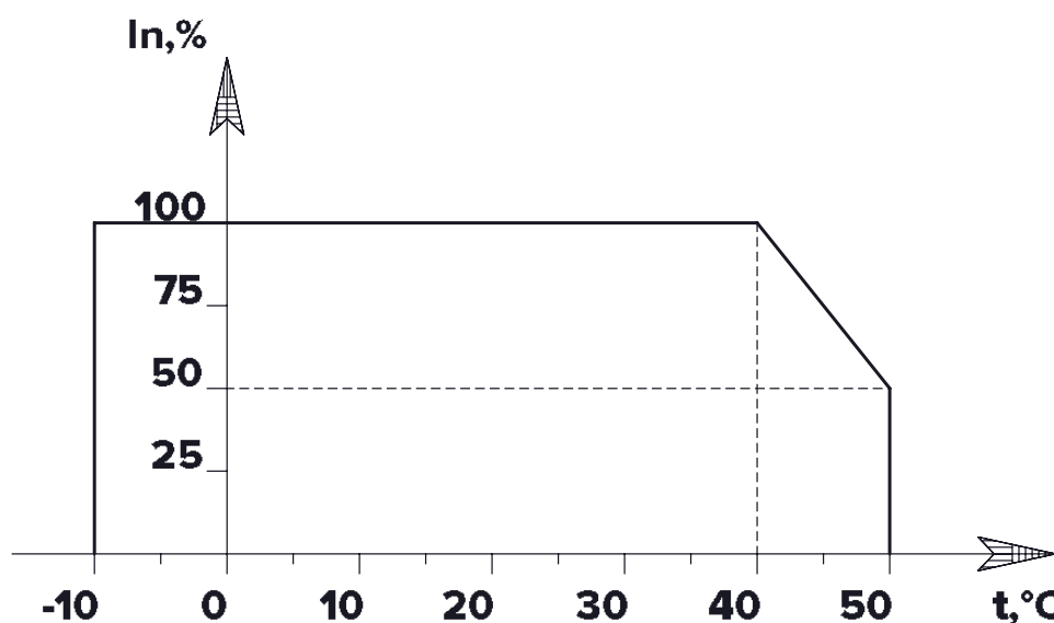
Рисунок 3.4—1 Снижение характеристики преобразователя частоты при превышении допустимой температуры
