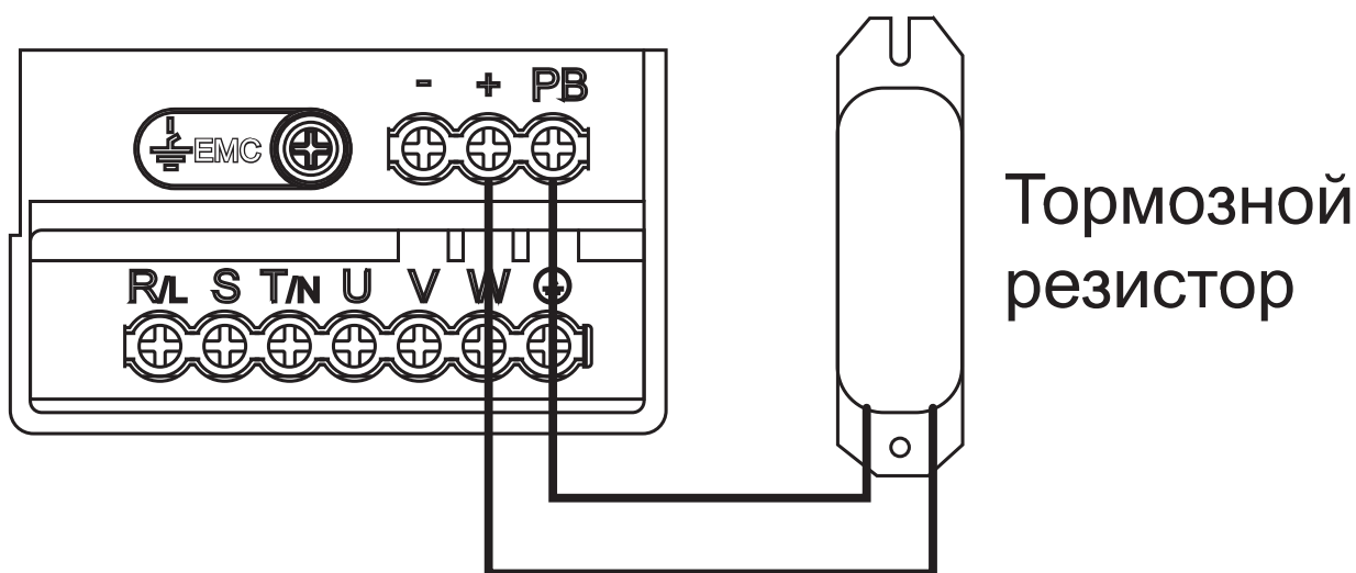
Рисунок 4.8-1 Подключение тормозного резистора для преобразователей частоты мощностью до 132 кВт (НП) (включительно) со встроенным тормозным ключом
