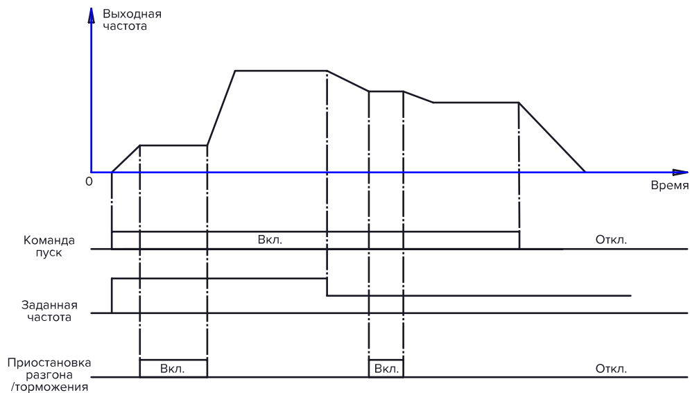
Рисунок 10.9-3 График приостановки разгона/торможения
