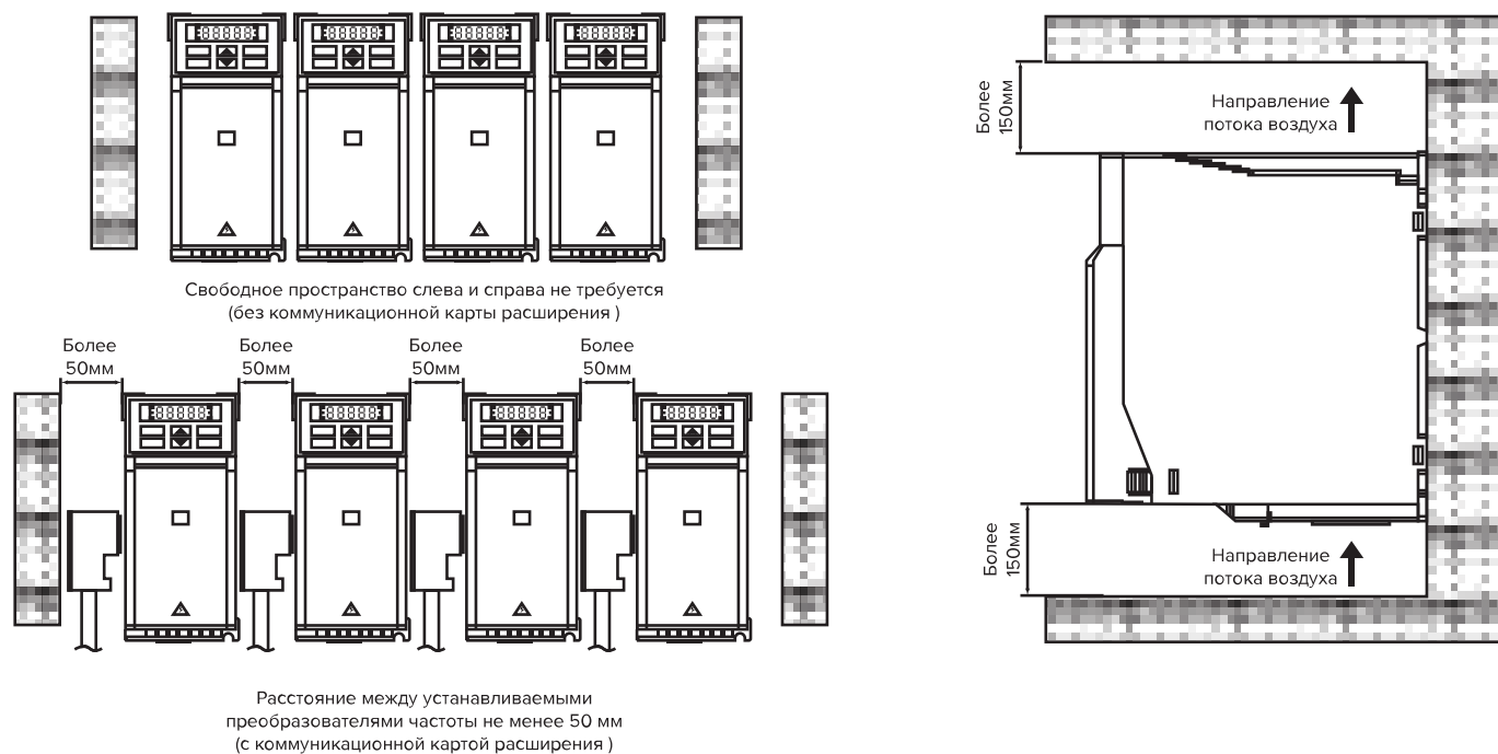
Рисунок 3.5—1 Положение преобразователя частоты и требуемое пространство
