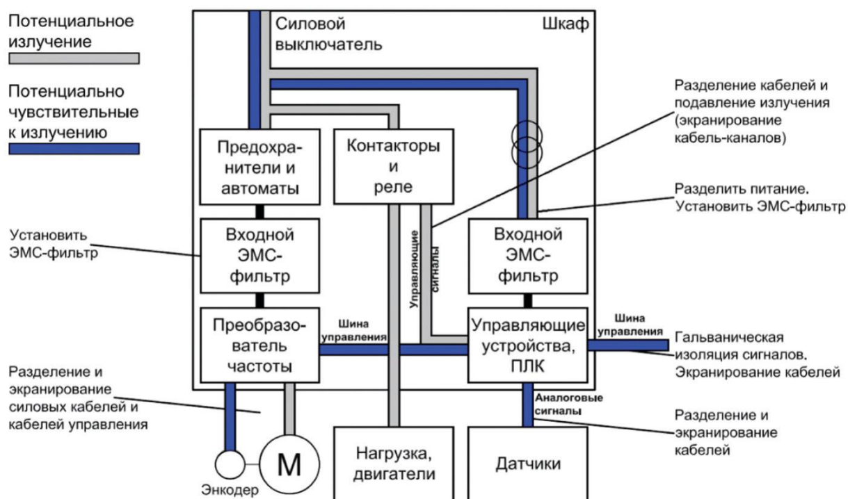
Рис. 4.10-1 План ЭМС на примере шкафа
