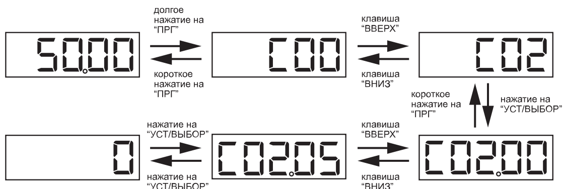
Рисунок 5.5-3 Основные операции на панели управления
