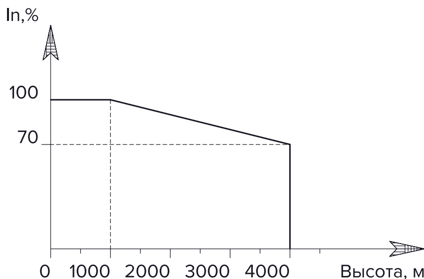
Рисунок 3.4—2 Снижение характеристики преобразователя частоты при превышении допустимой высоты
