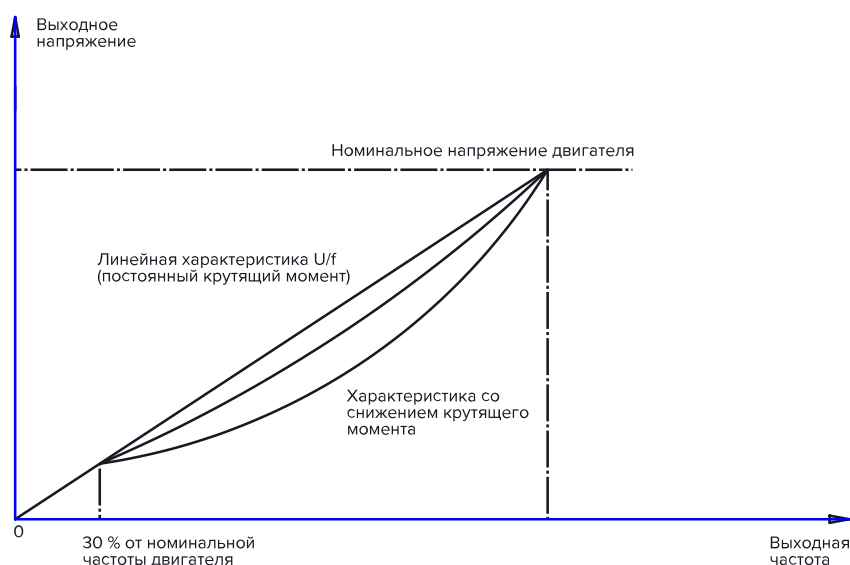
Рисунок 10.8-1 Усиление крутящего момента
