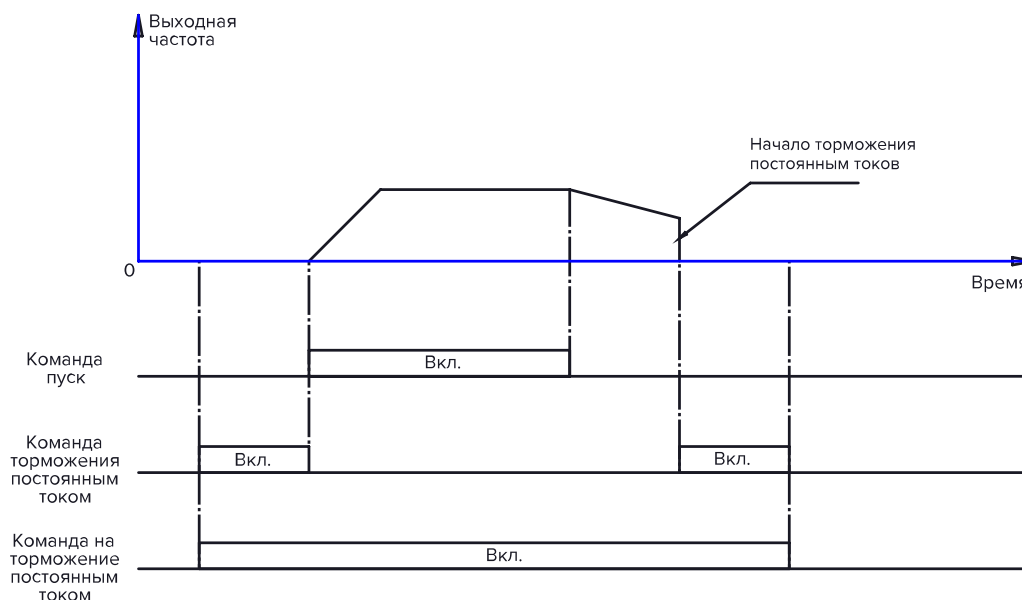
Рисунок 10.9-4 График торможения постоянным током
