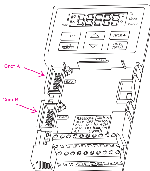
Рисунок 6.2-1 Расположение слотов (разъемов) на передней части преобразователя частоты
