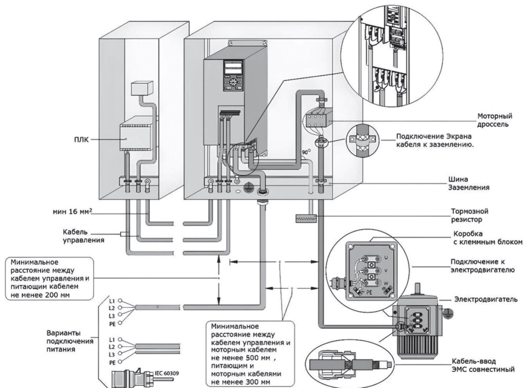
Рис. 4-10-2 Пример выполнения электрического монтажа преобразователя частоты со степенью защиты IP20 с учётом требований ЭМС
