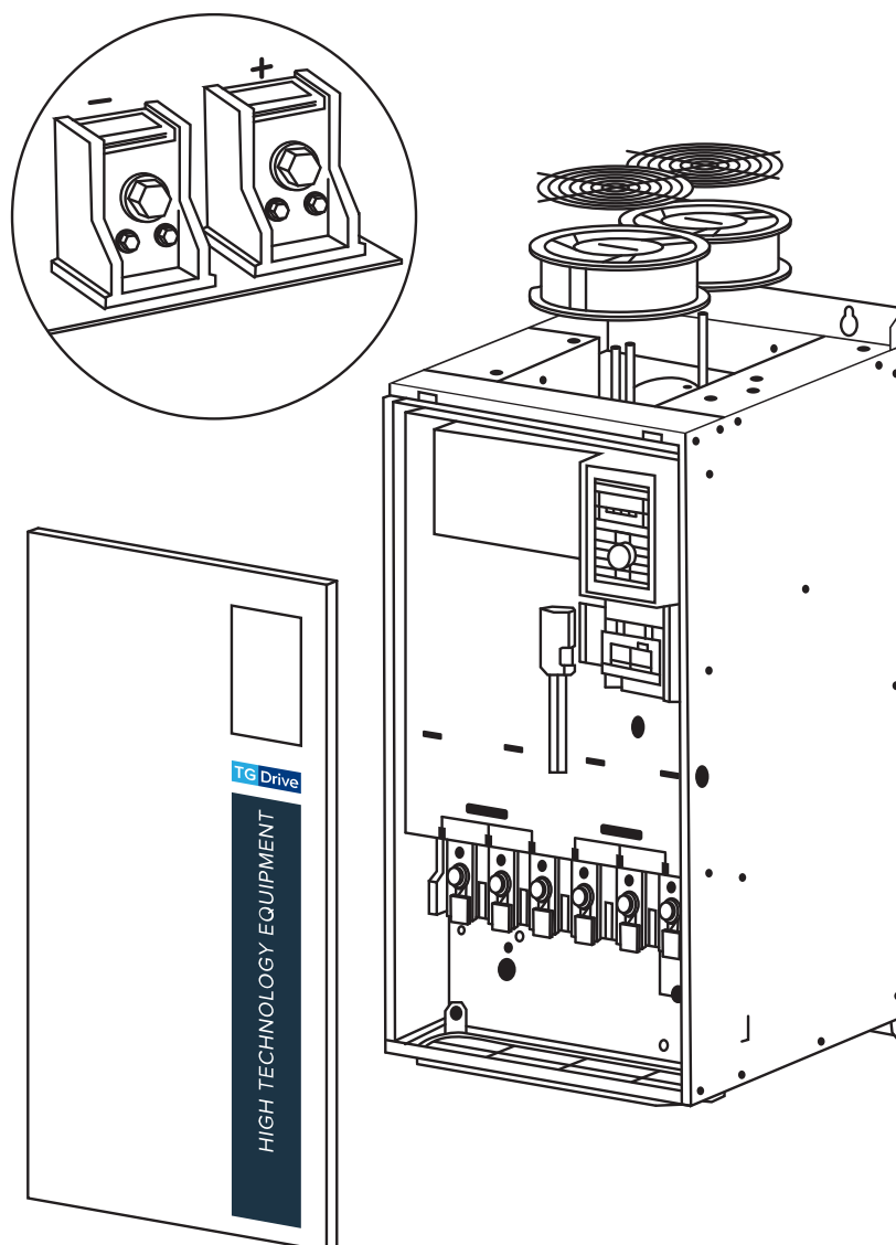
Рисунок 4.4-2 Конструкция преобразователя частоты с металлическим корпусом серии TG910
