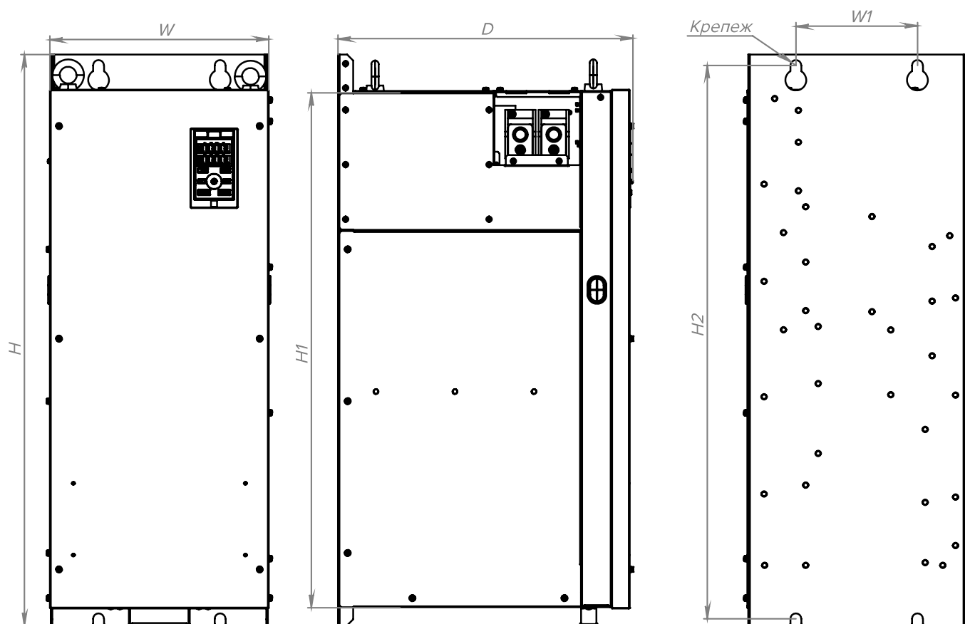
Рисунок 3.6-9 Чертеж преобразователя частоты типоразмер C01
