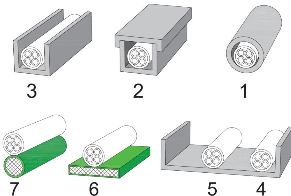
Рисунок 4.10-3. – Примеры прокладки неэкранированных моторных кабелей для уменьшения шумов (помех) выходных сигналов:
