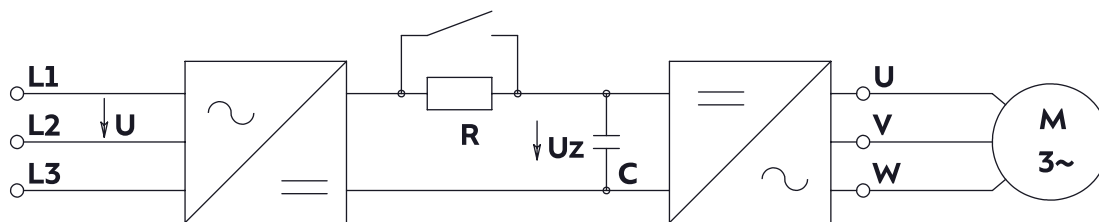
Рисунок 1.5–1 Схема силовой части преобразователя частоты с промежуточным звеном постоянного тока
