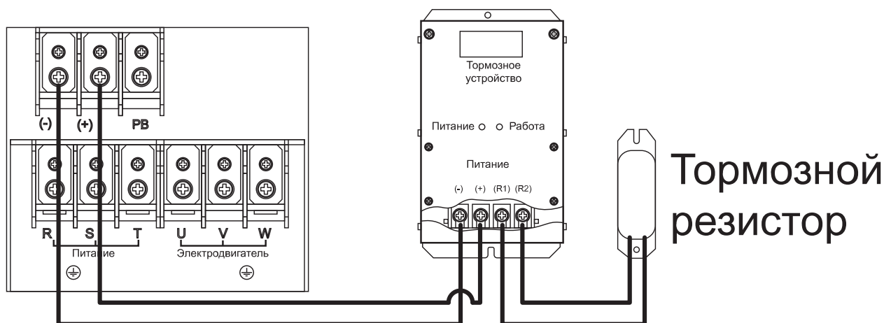
Рисунок 4.8-2 Подключение тормозного резистора для преобразователей частоты через внешний тормозной модуль
