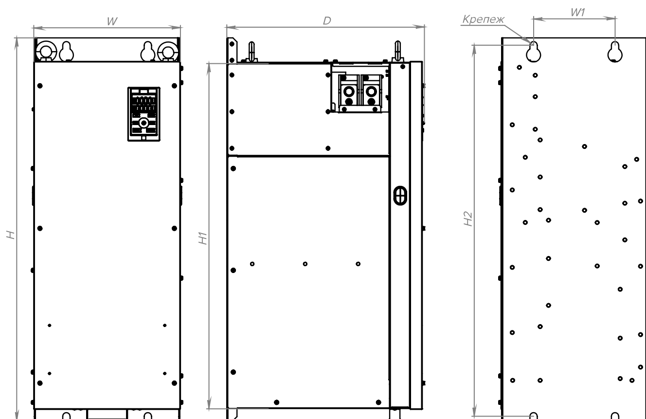
Рисунок 3.6-11 Чертеж преобразователя частоты типоразмер С03
