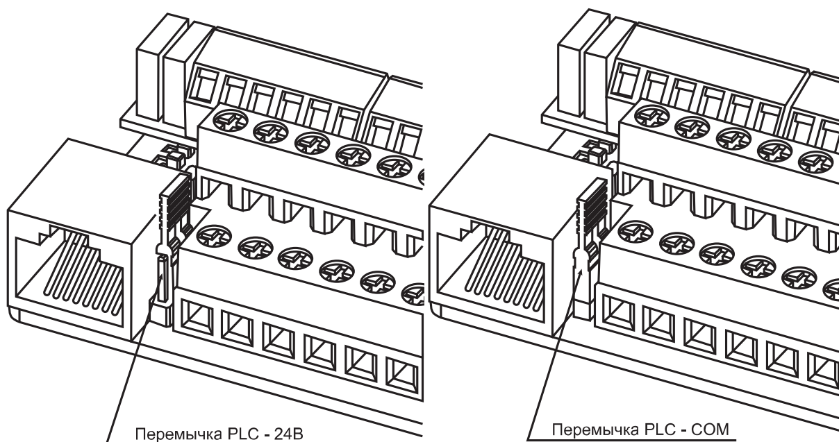
Рисунок 4.7-3 Схема подключения перемычек «+24В», «PLC», «COM»
