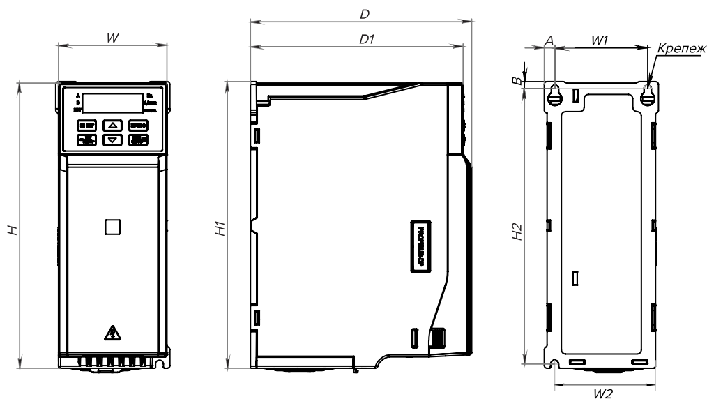
Рисунок 3.6—1 Чертеж преобразователя частоты типоразмер А01
